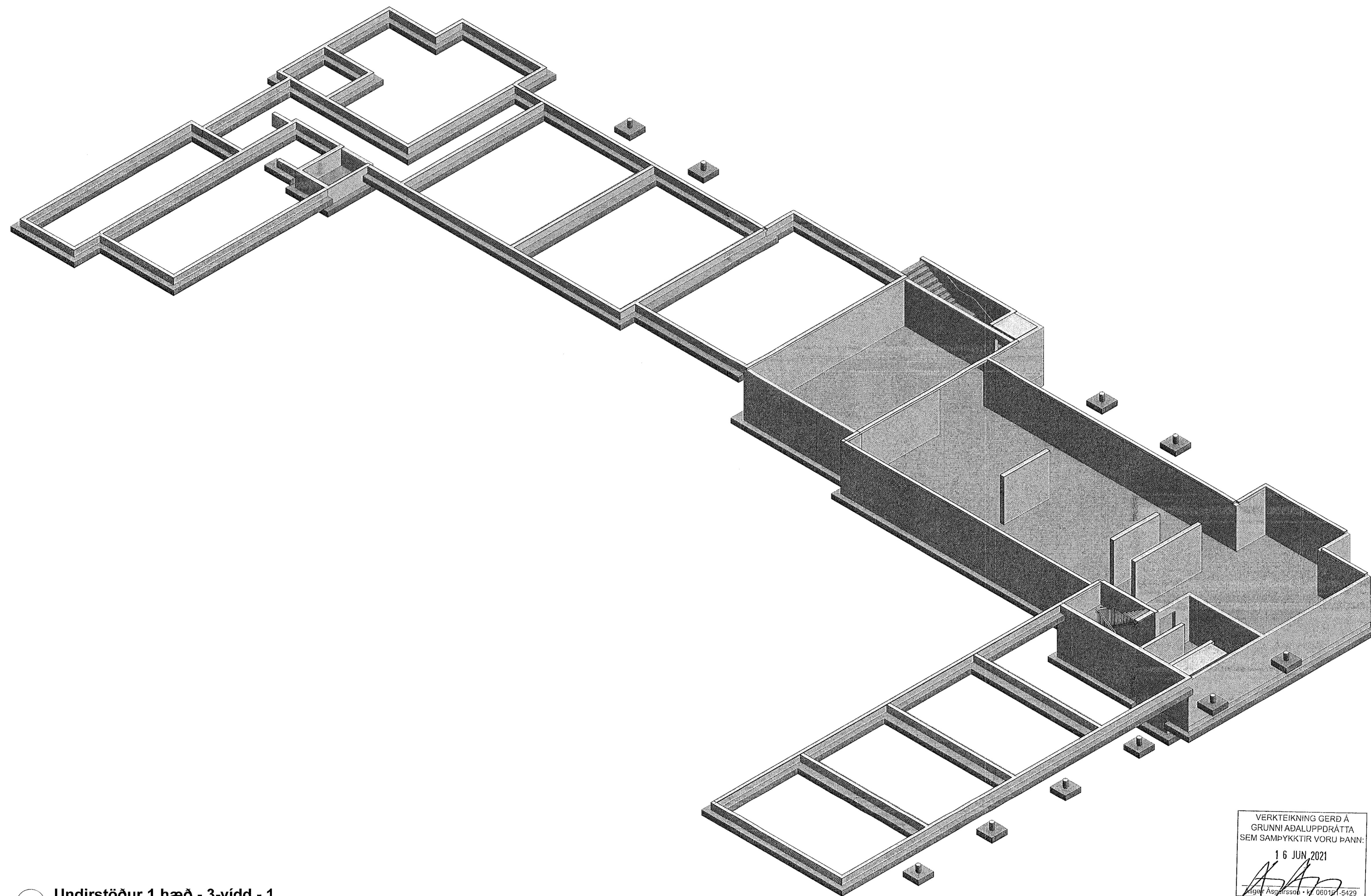
1 Undirstöður 1.hæð - 3-vidd - 1
