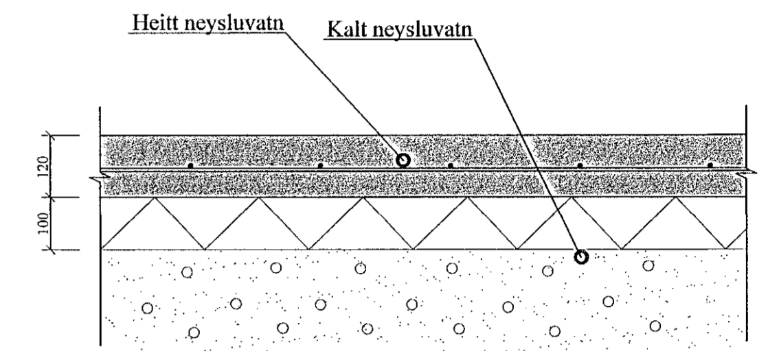
SNIÐ Í LÖGN. 1:10
