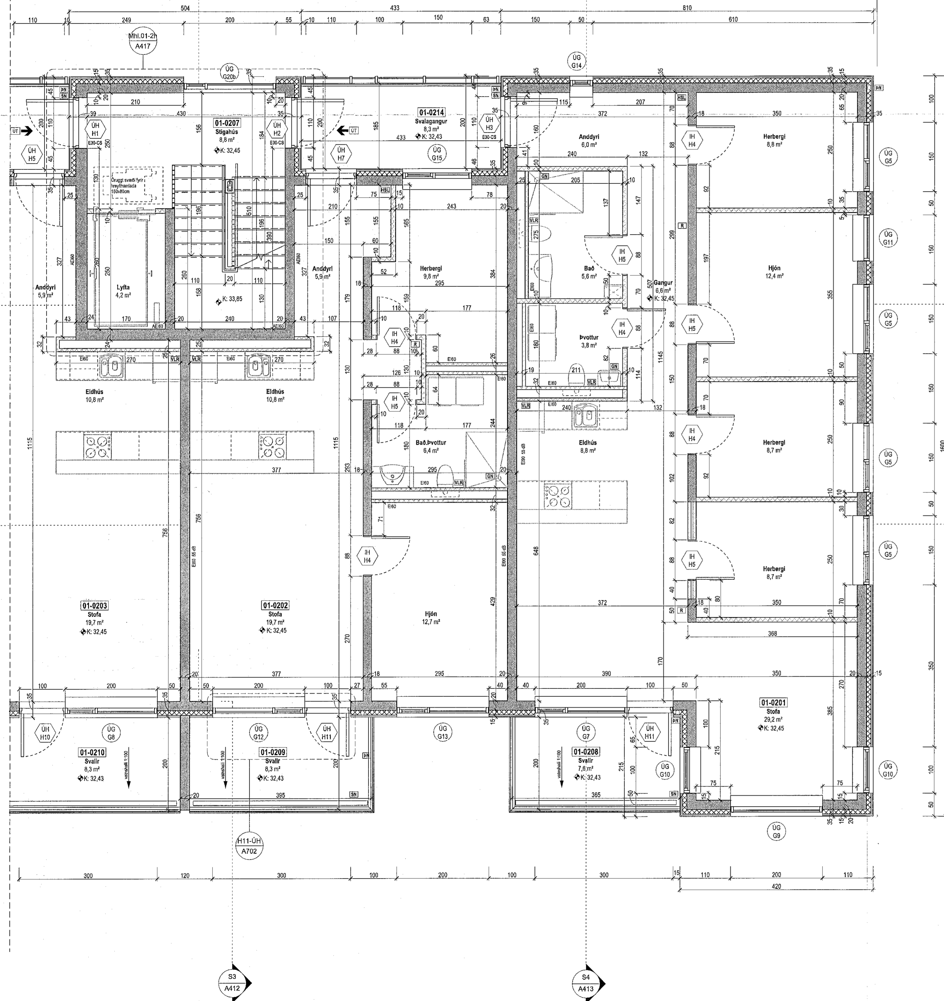
Grunnmynd 2.hæð 1:50
