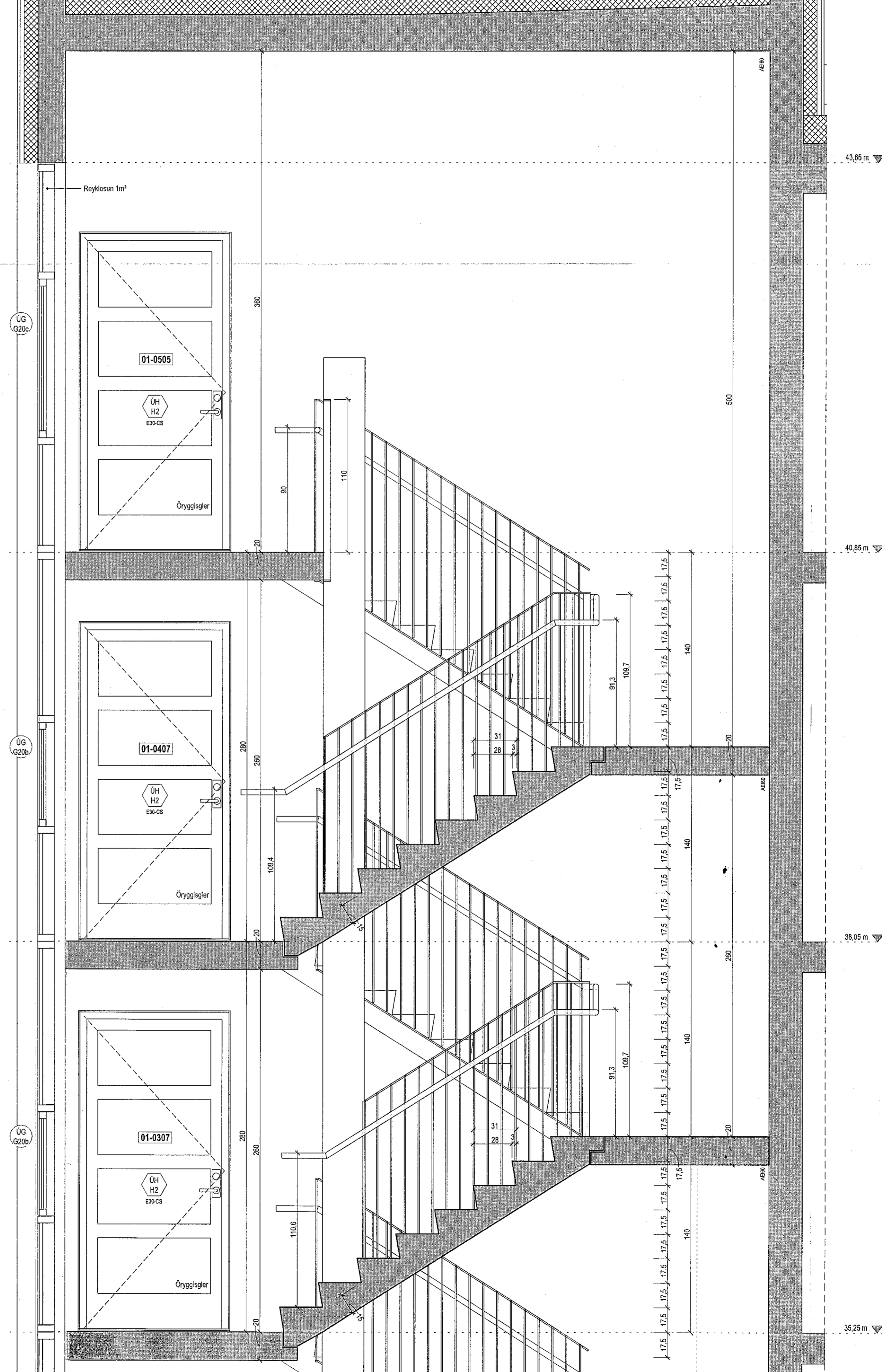
Snið 7b 1:20
