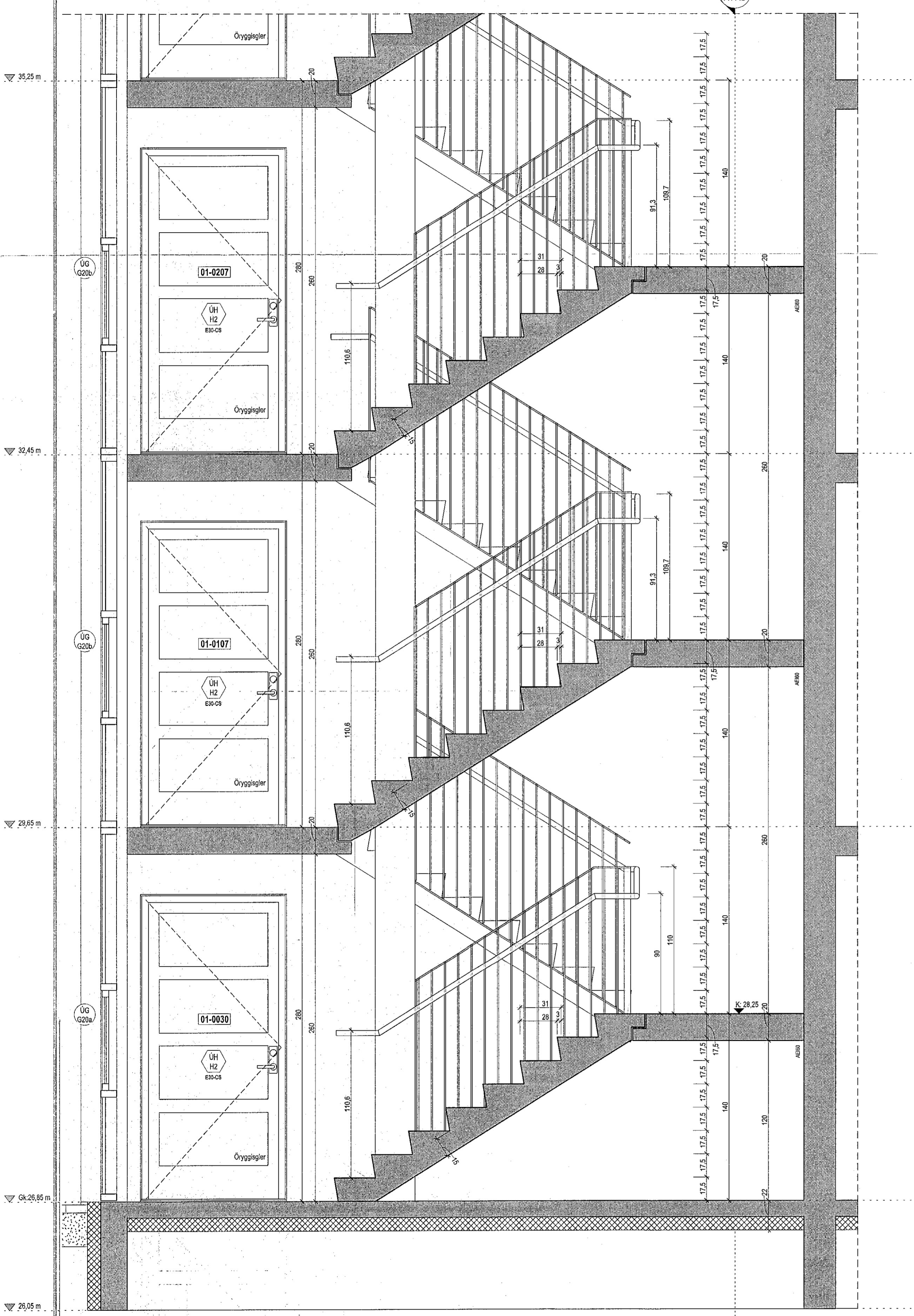
Snið 7a 1:20
