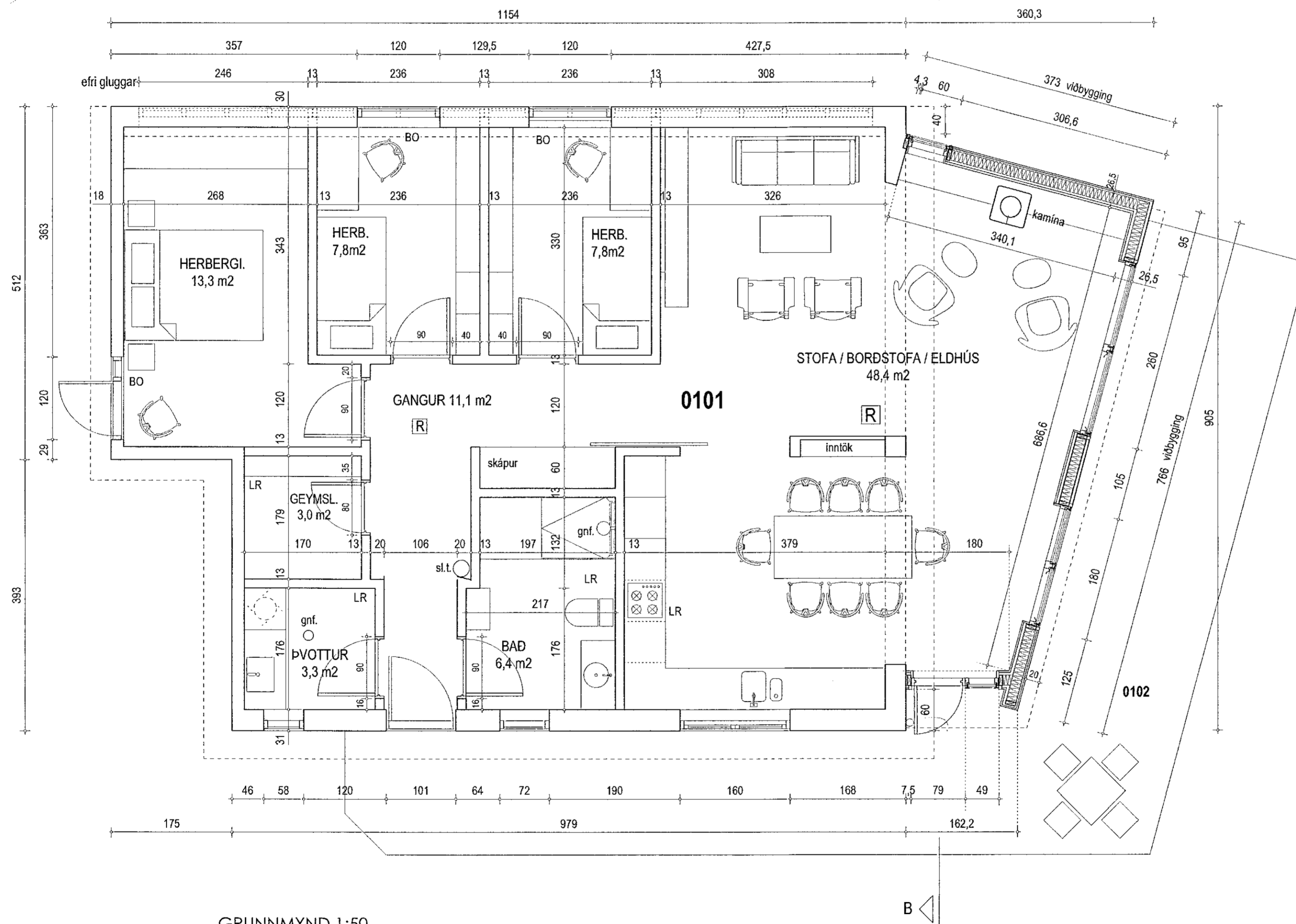
GRUNNMYND 1:50
