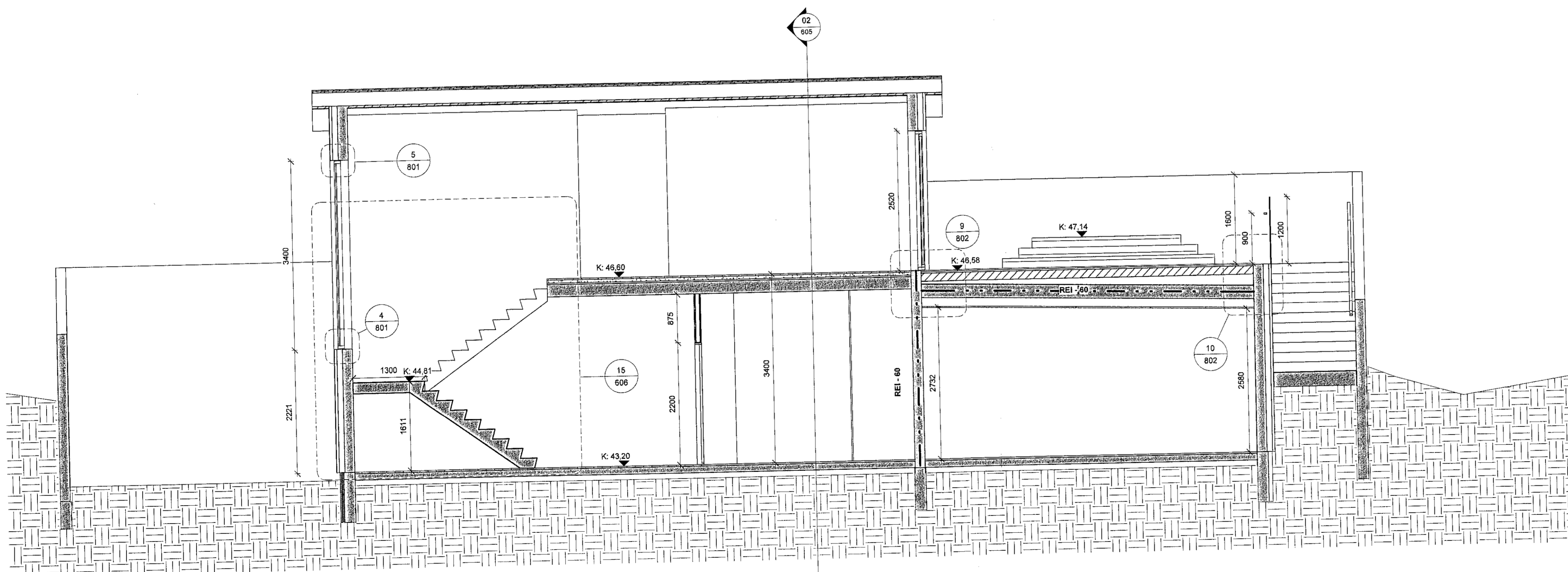
01 Verkteikning - Snið 01 1:50
