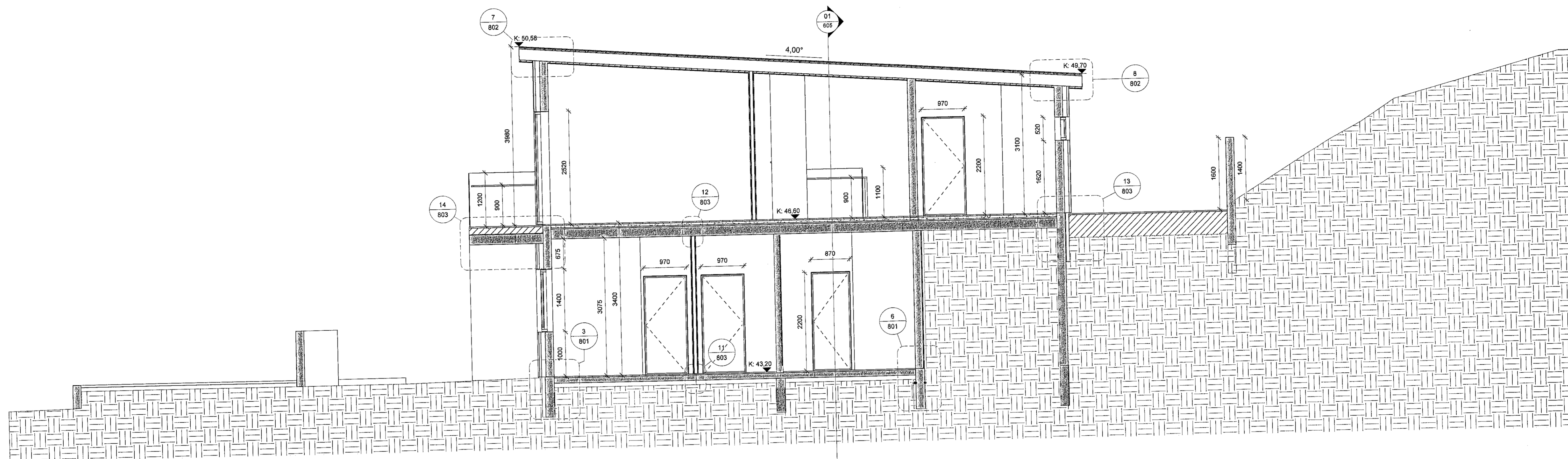
02 Verkteikning - Snið 02 1:50
