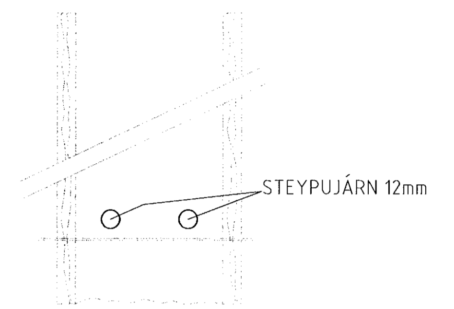
SNID AF STEYPUVEINUM Í SÖKKLUM ENGINN MÆLIKVARDI
