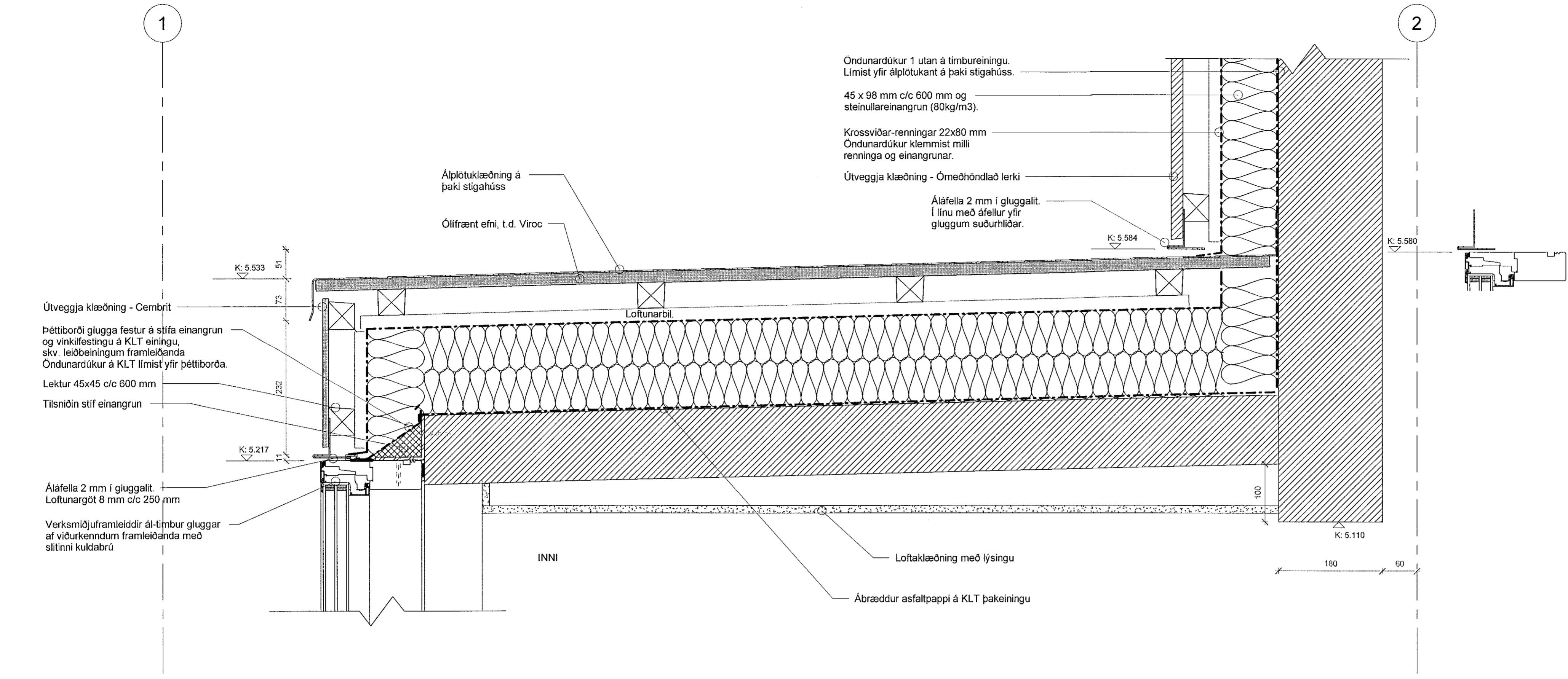
2 Lóðrétt deili þak stigah 1:5
