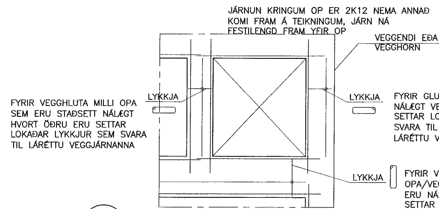
K0 ASÝND Á VEGG - JÁRNUN VEGGHLUTA Mkv. 2
