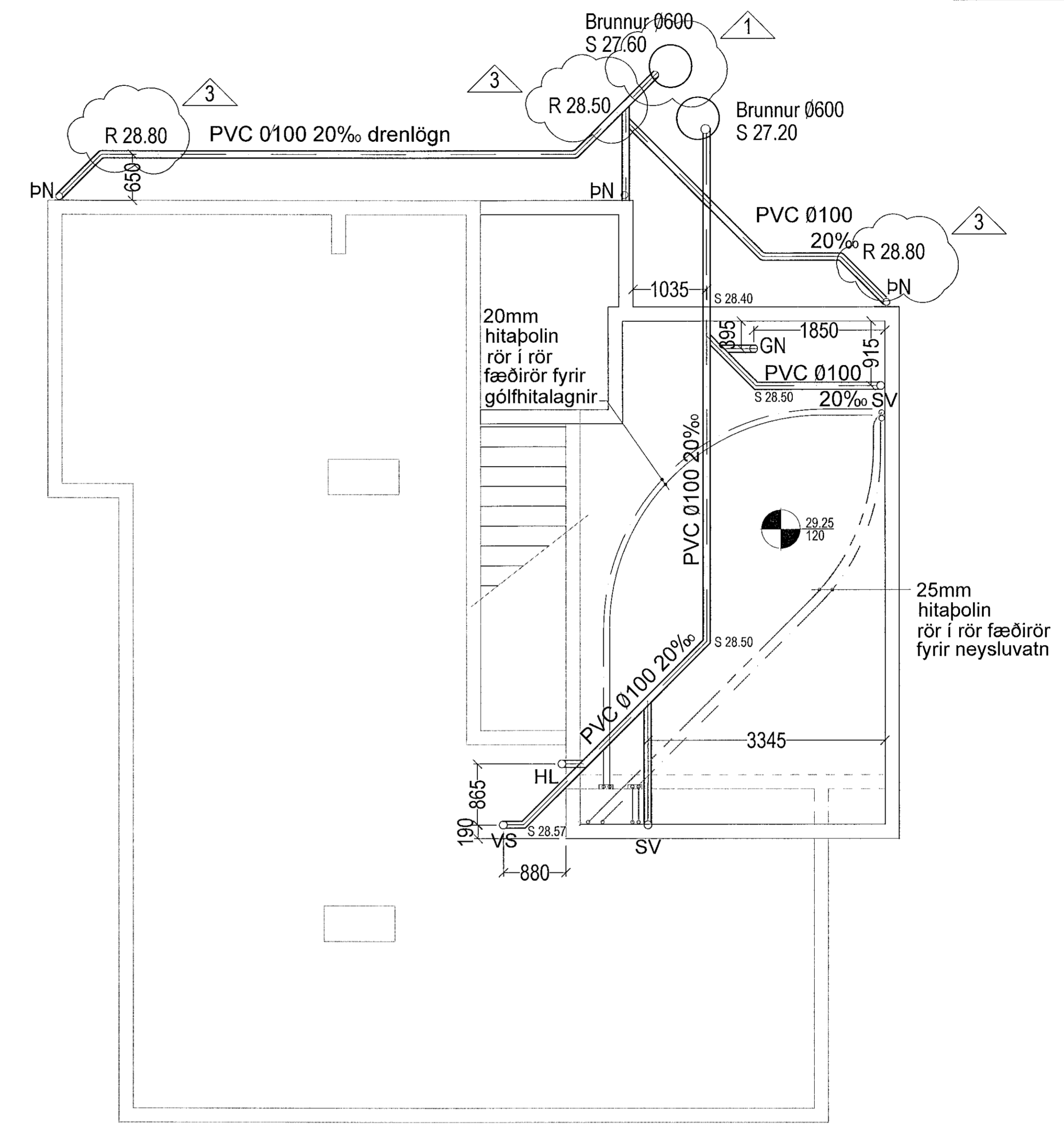
Grunnmynd Mkv. 1:50
