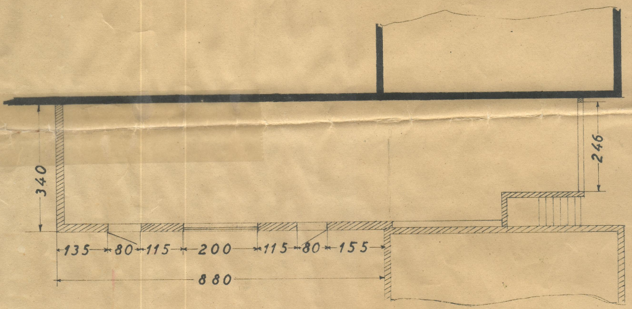
Grunnmynd.
