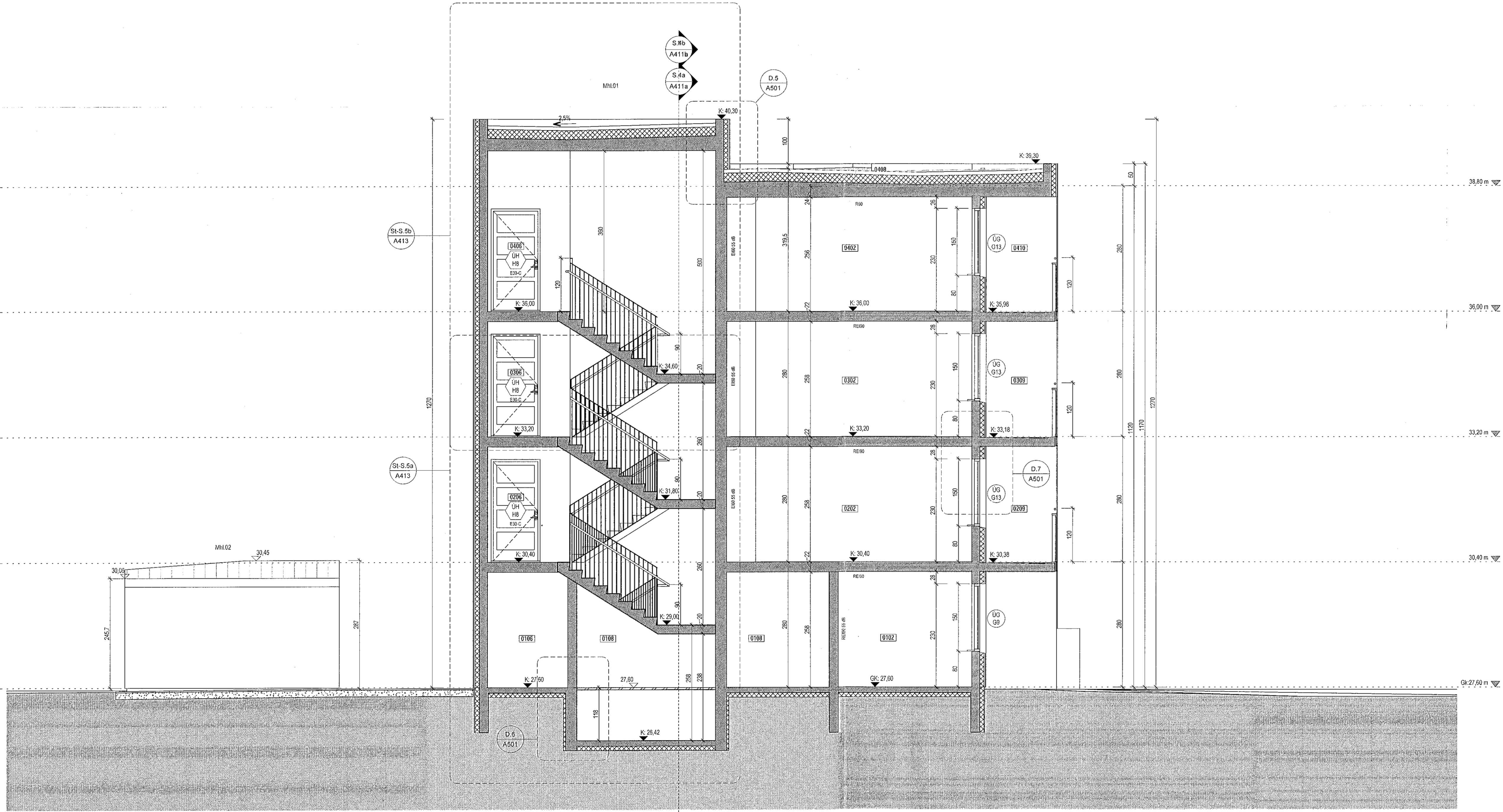
Snið 2 1:50
