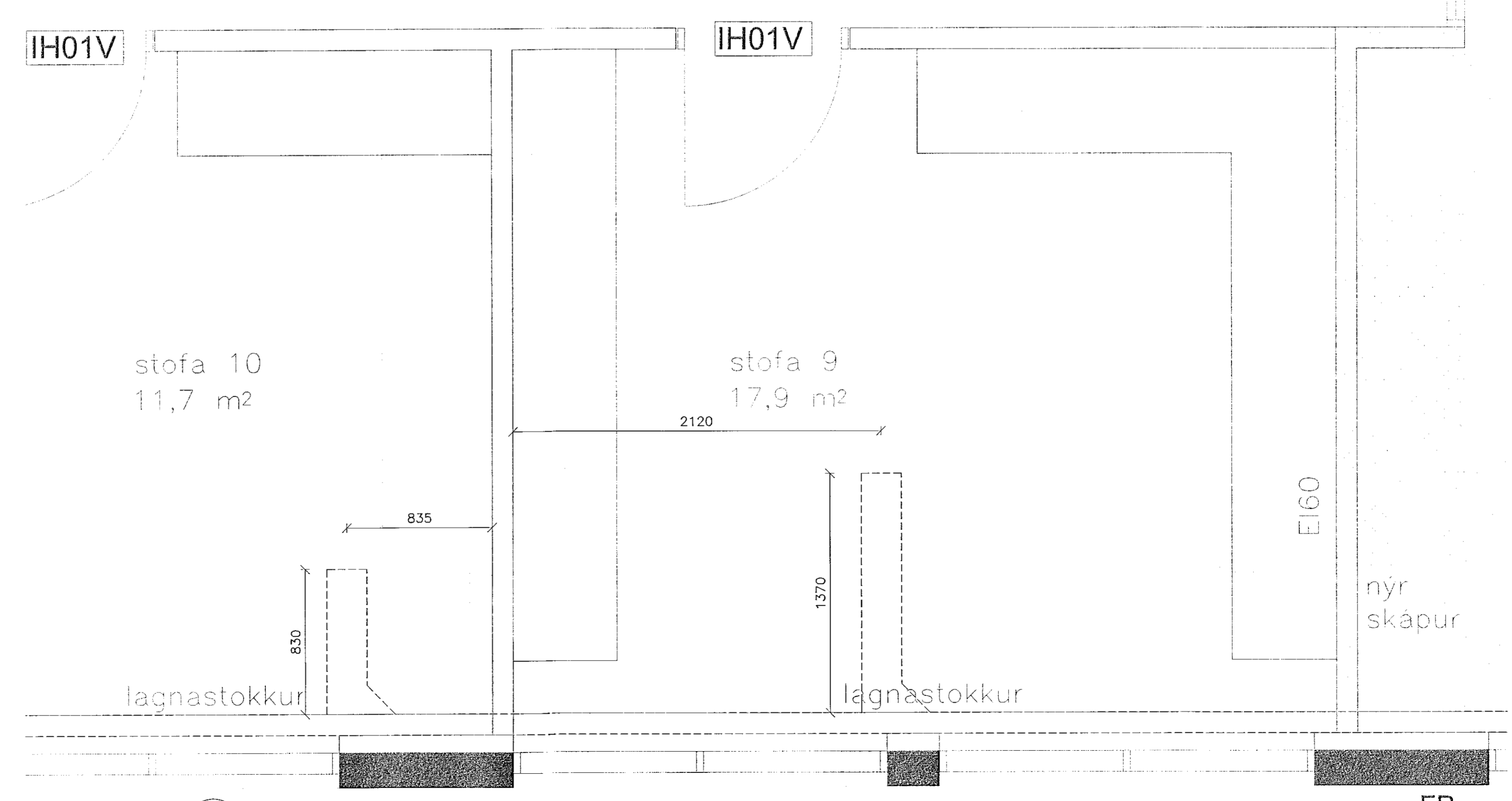
2 Grunnmynd, 2 hæð Mkv: 1:20
