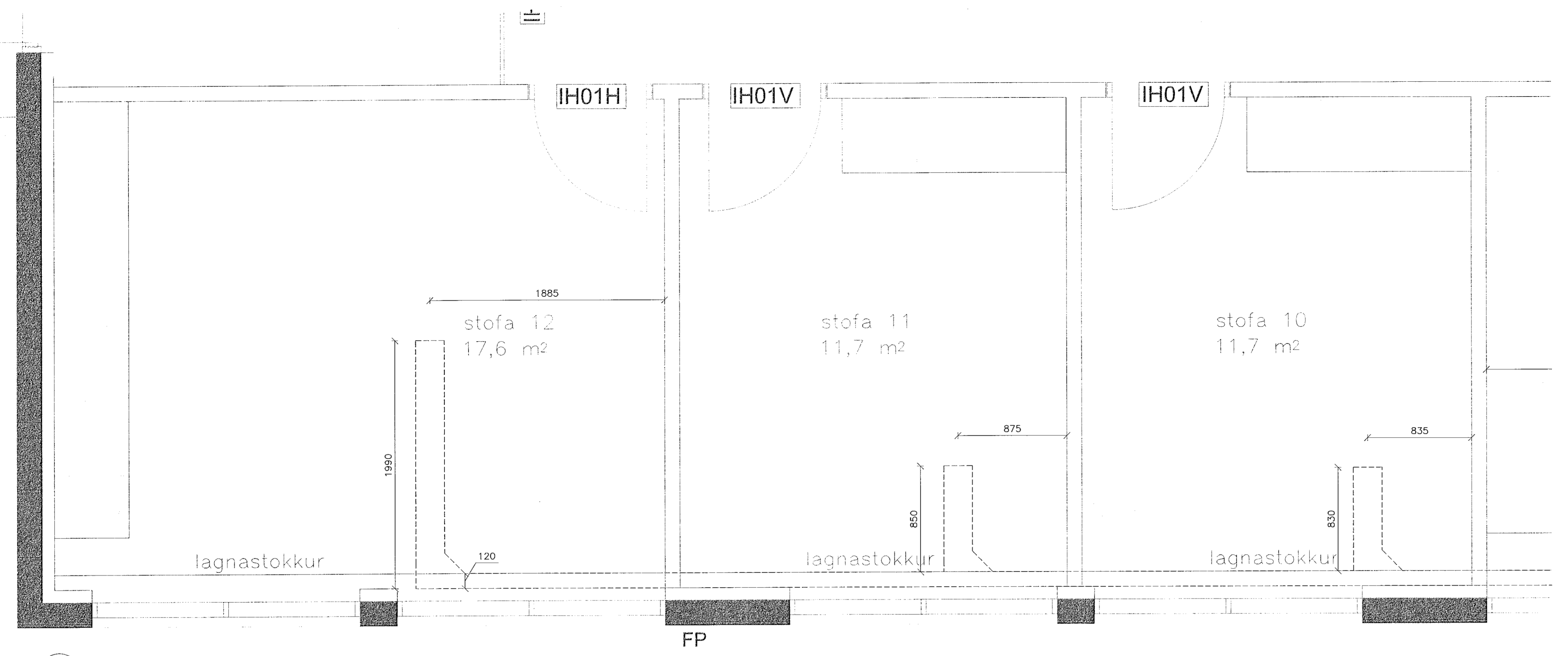
1 Grunnmynd, 2 hæð Mkv: 1:20
