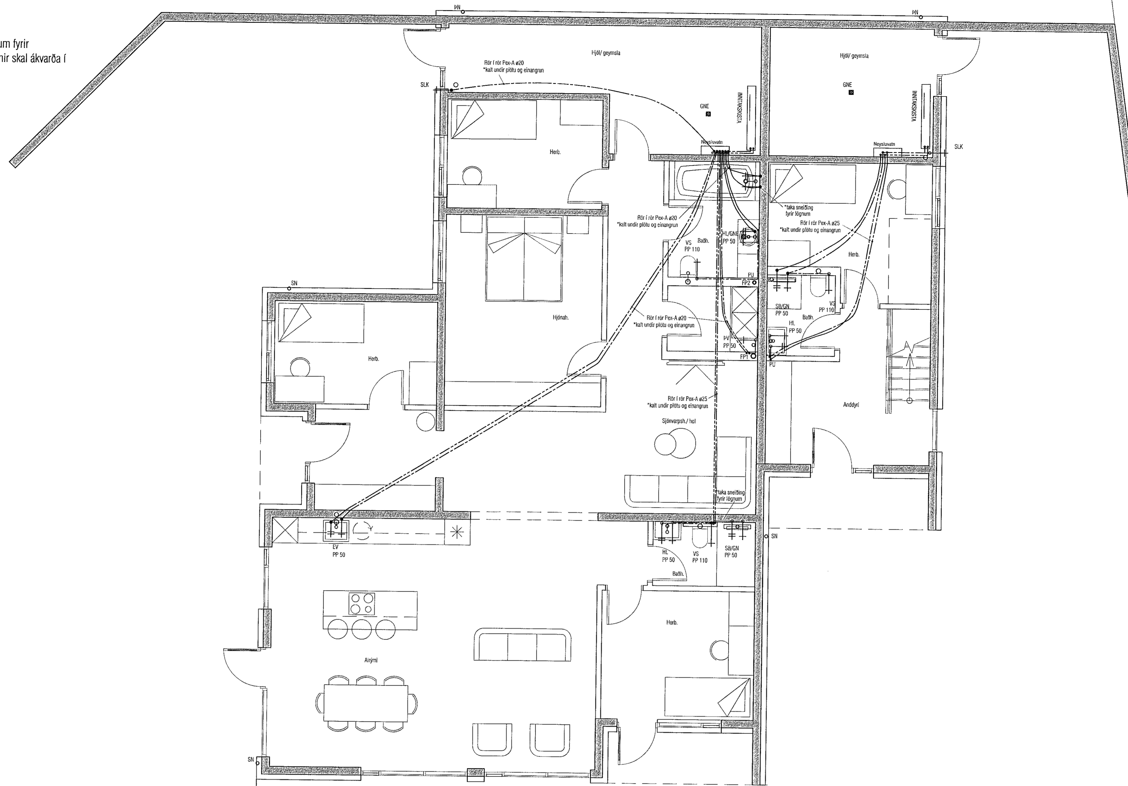
GRUNNMYND ÞRIFALAGNA 1.HÆÐ
