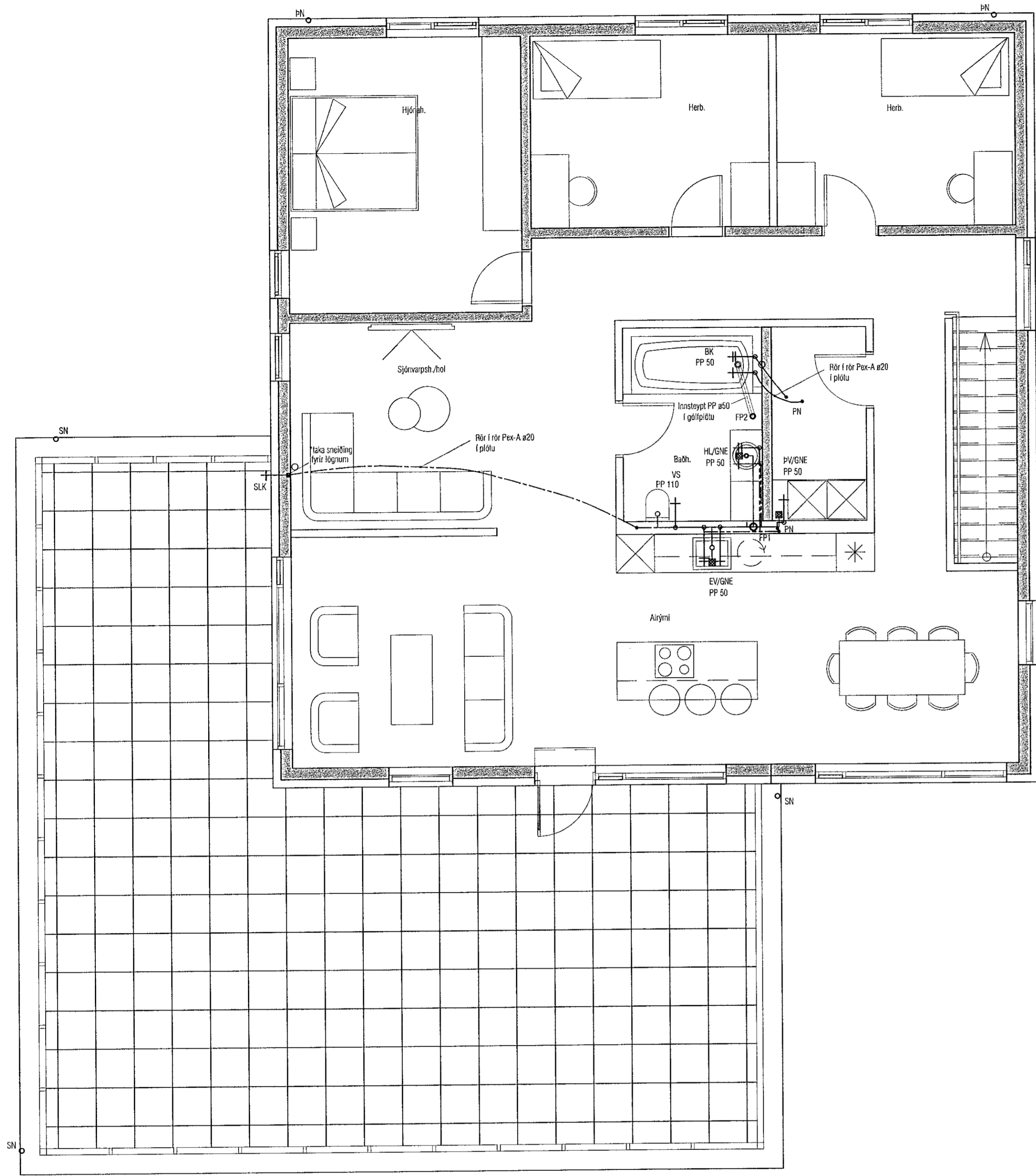
GRUNNMYND ÞRIFALAGNA 2.HÆÐ
