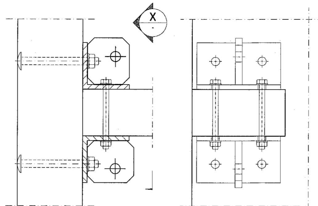
B1 Mkv. 1:5 Boltast saman með: 4 stk. borðboltum M16x180 2 stk. stálboltum M16x150
