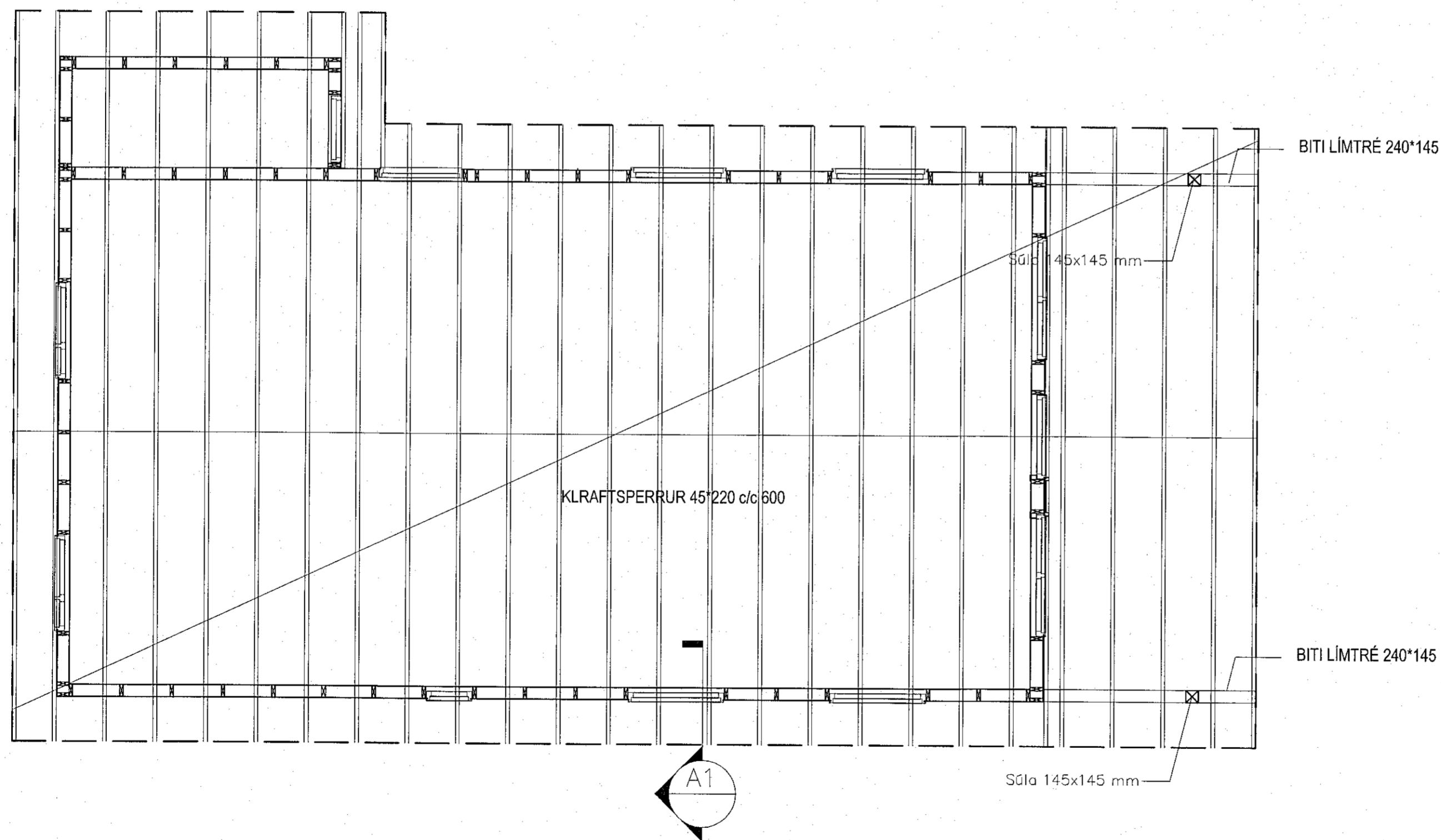
ÞAKVIRKI GRUNNMYND. mkv. 1 : 50.
