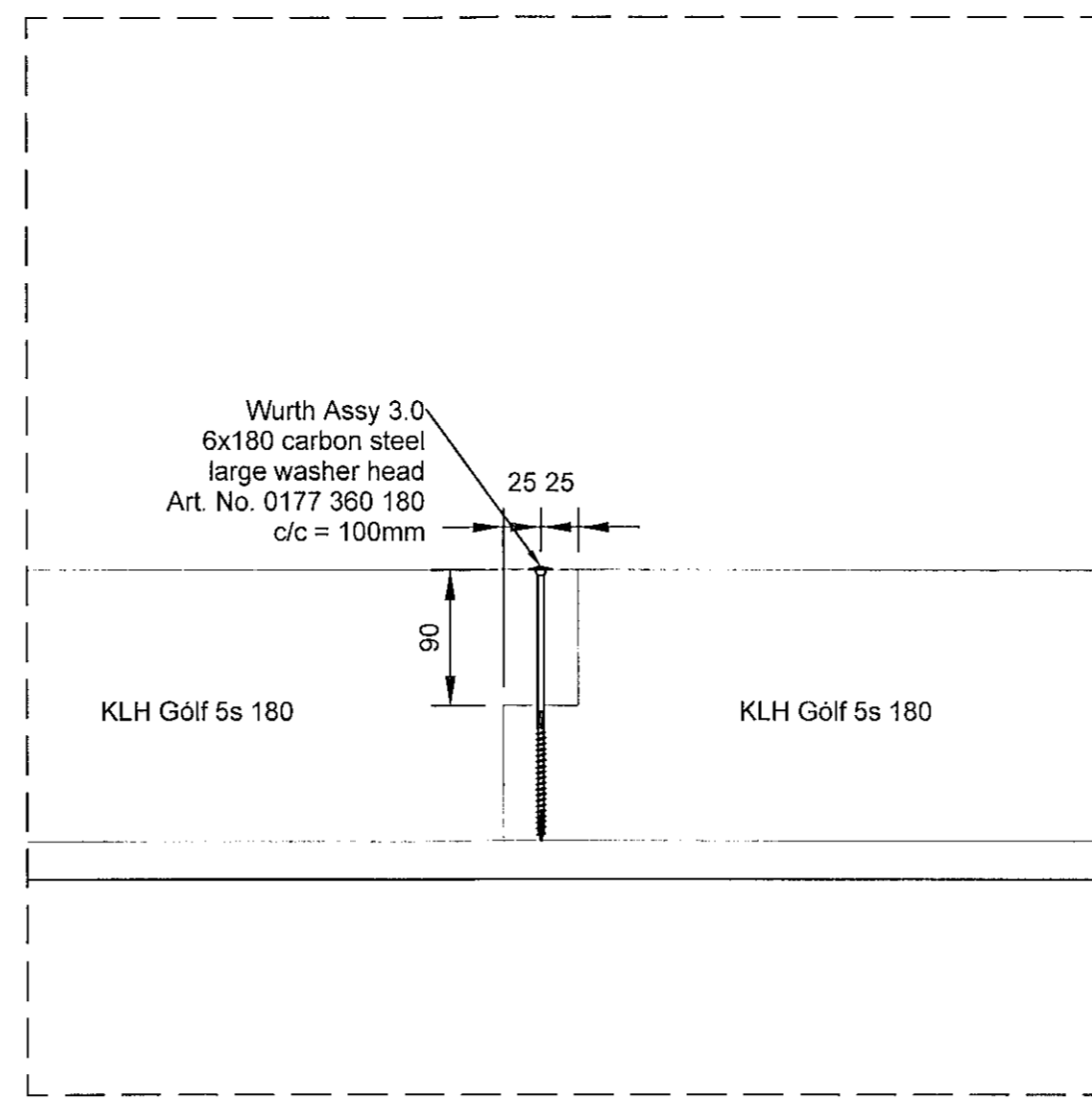
Deili C3 1:5
