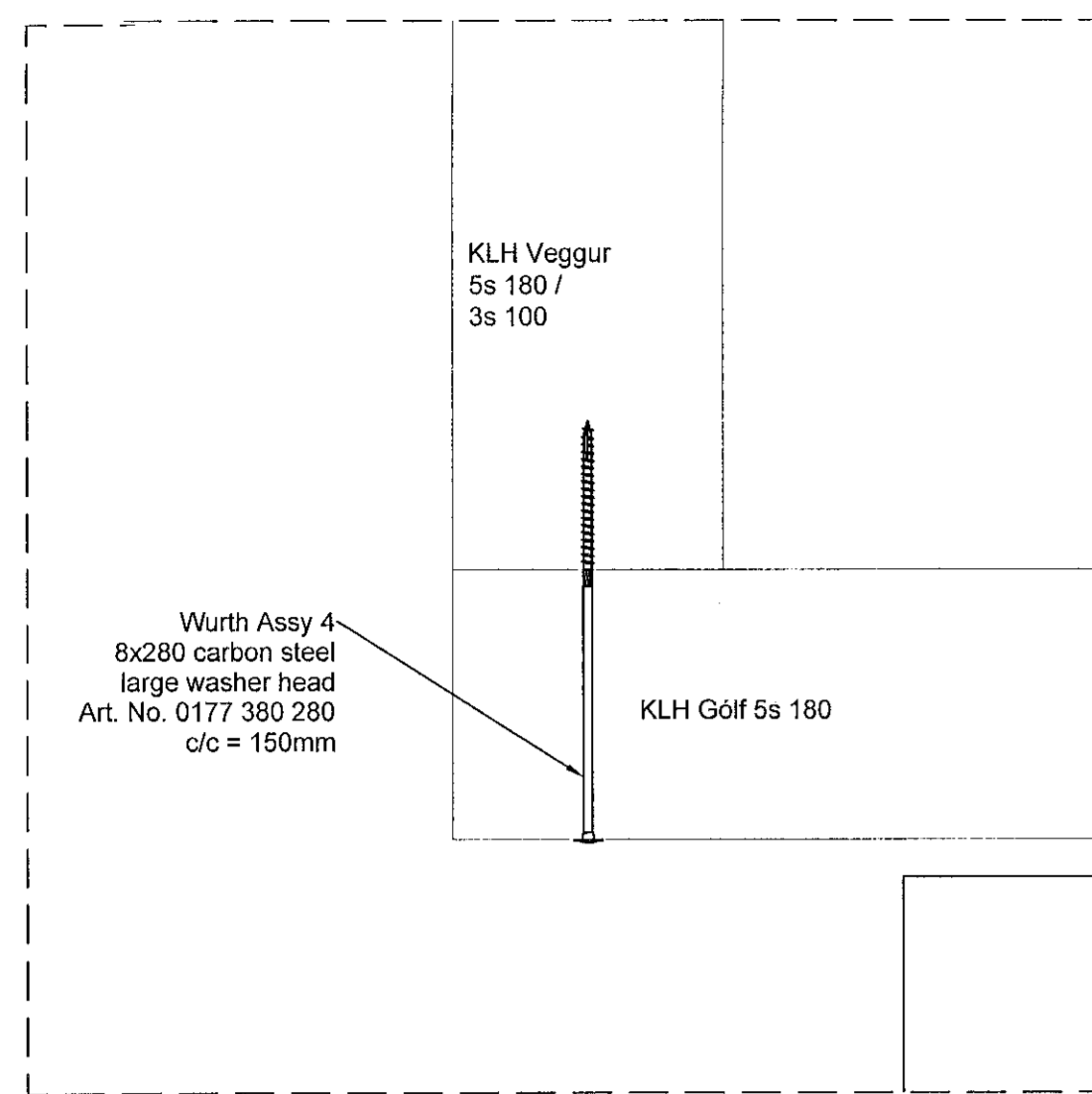
Deili C1 1:5
