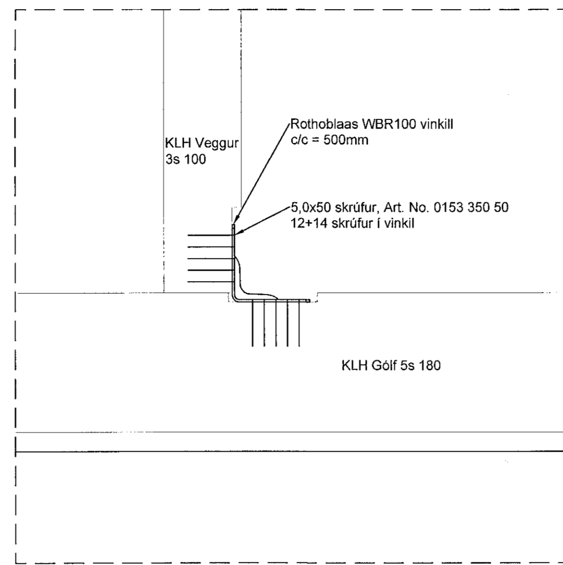
Deili C2 1:5
