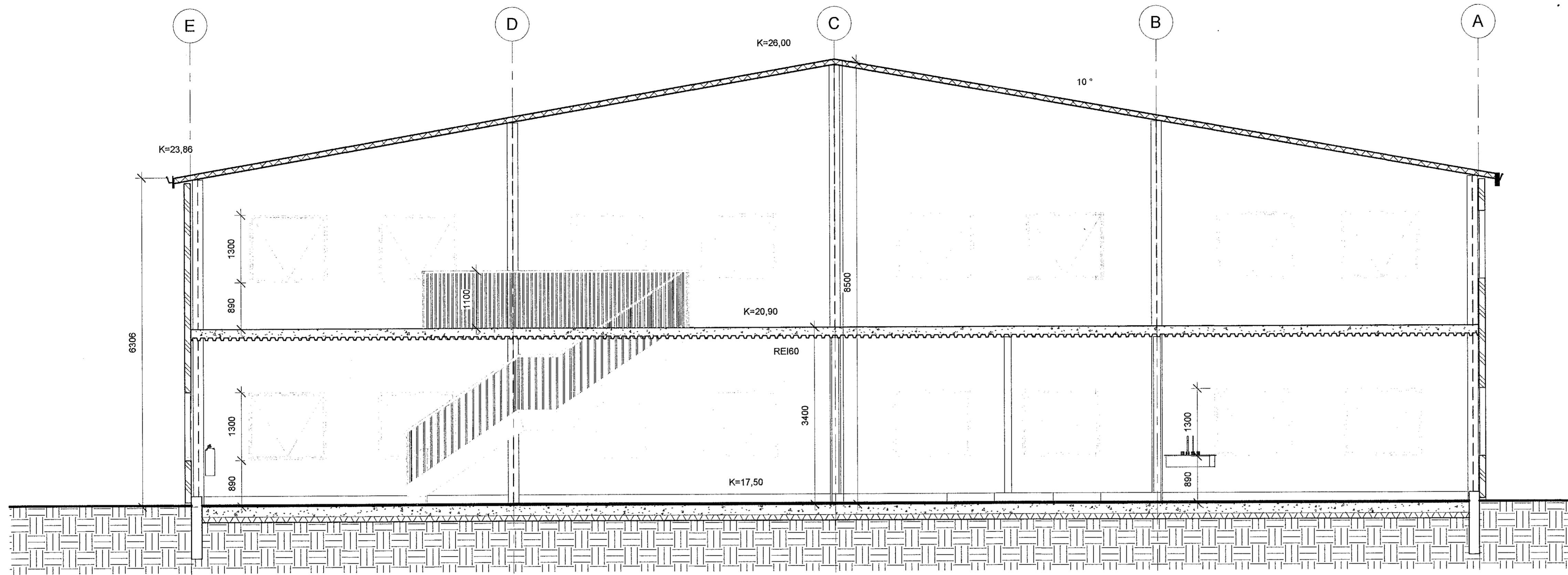
1 Snið 1 1-50 1 : 50
