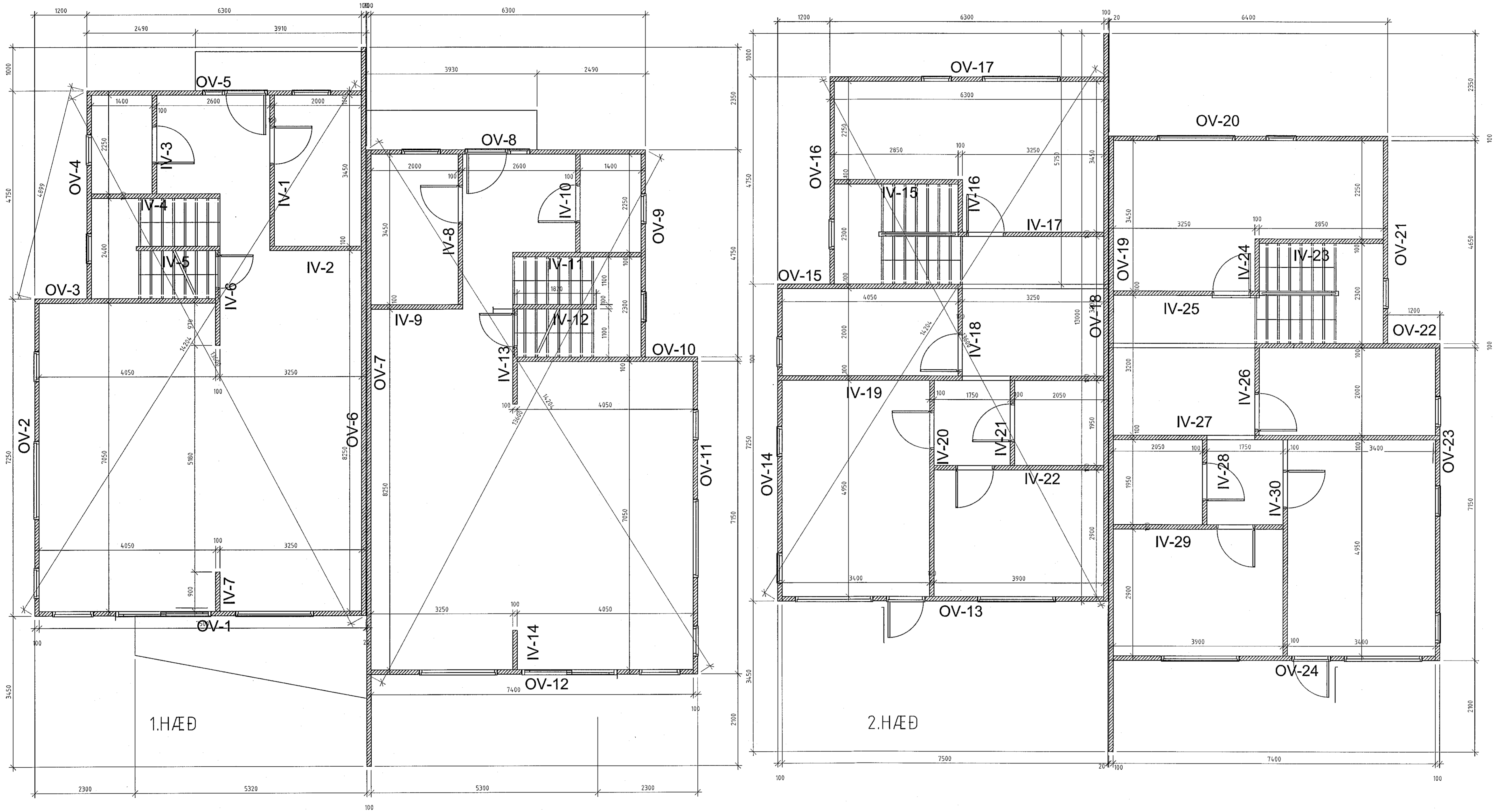
GRUNNMYND HÆÐA1:50
