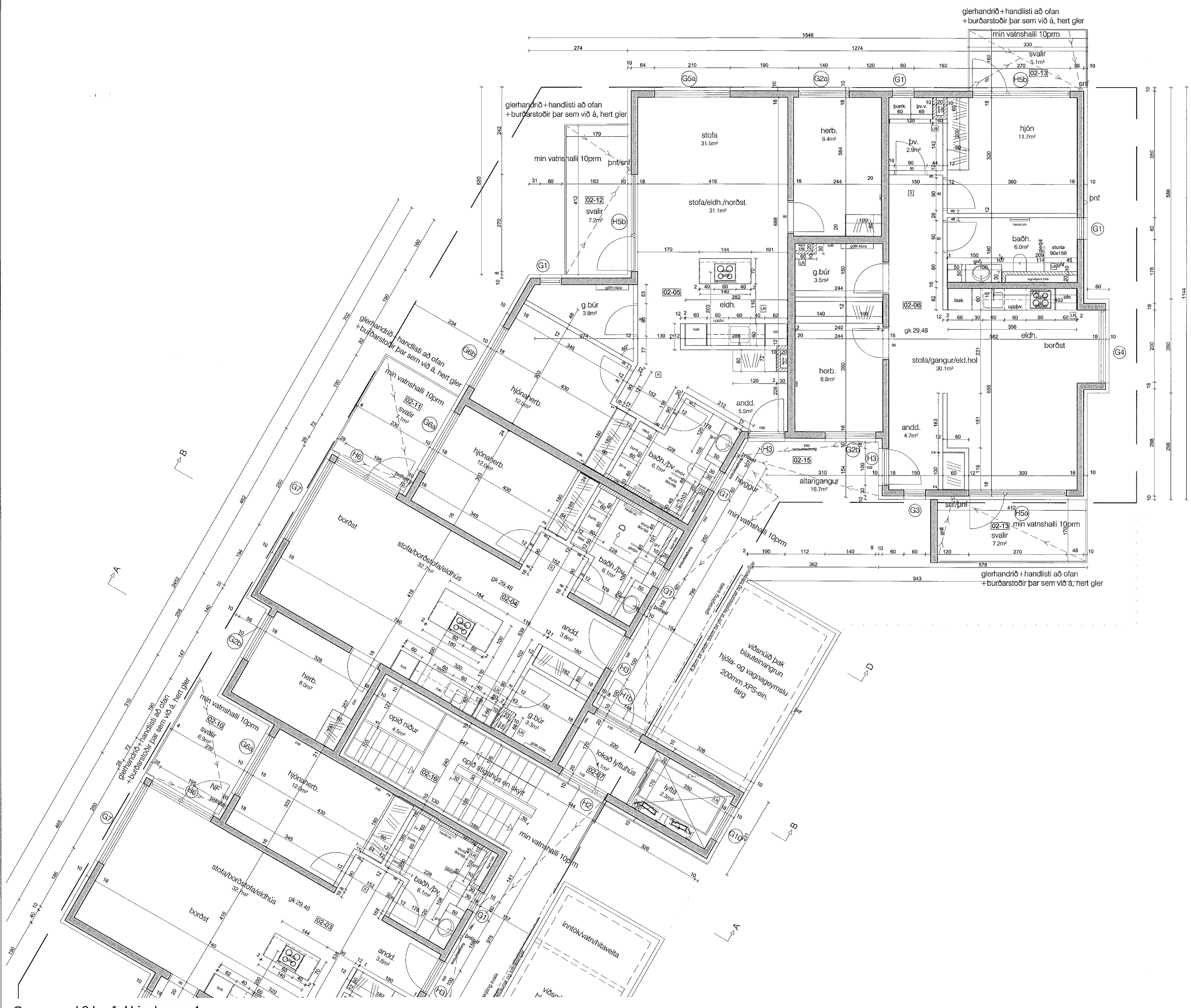
Grunnmynd 2.hæð, Hringhamar 1
