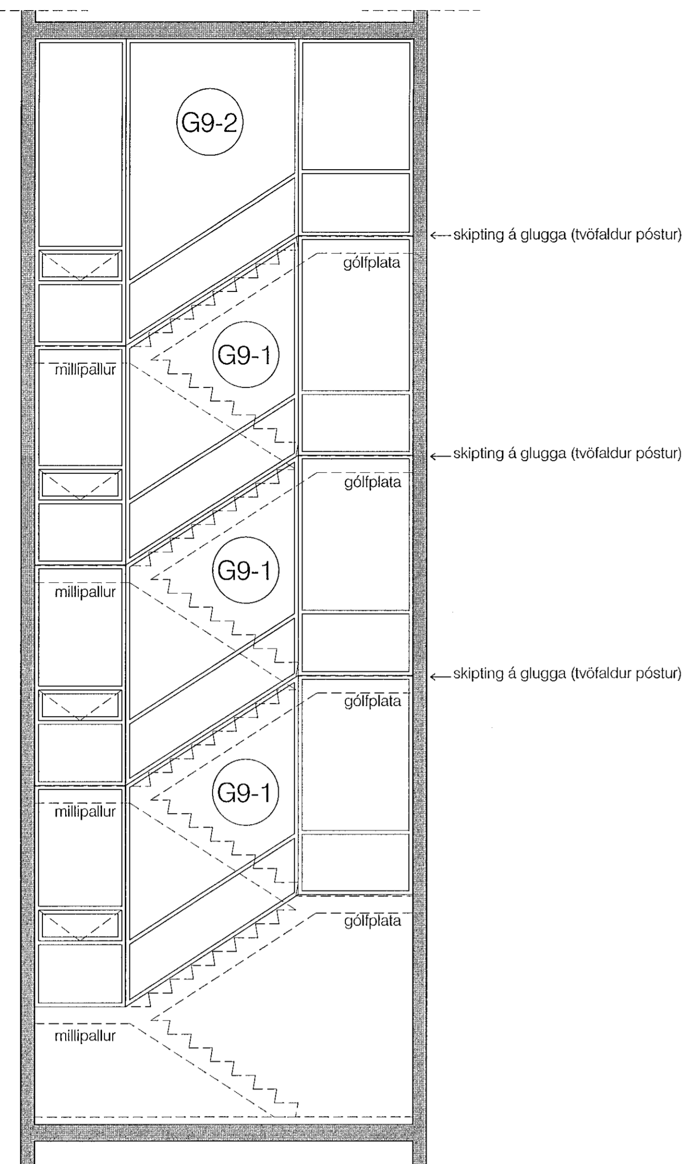
yfirlitsmynd: G9-1, G9-2
