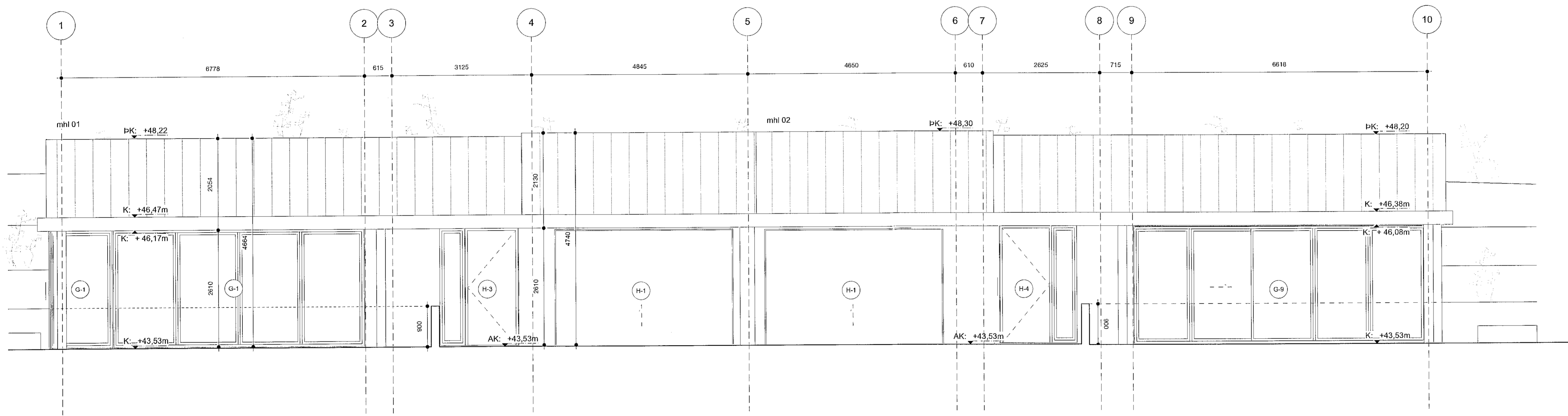
Ásýnd vestur mkv: 1:50
