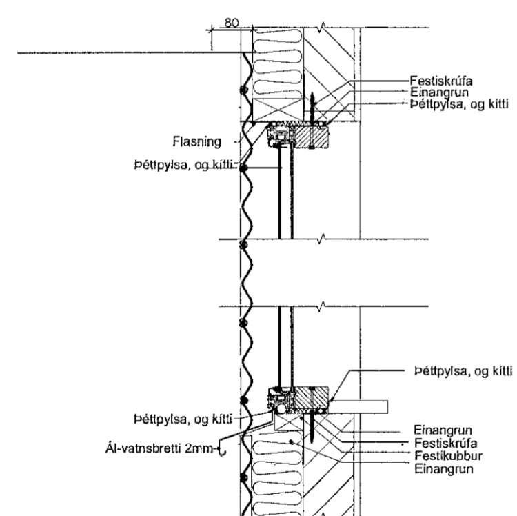
Ísetning glugga, Lóðréttur skurður 1:10
