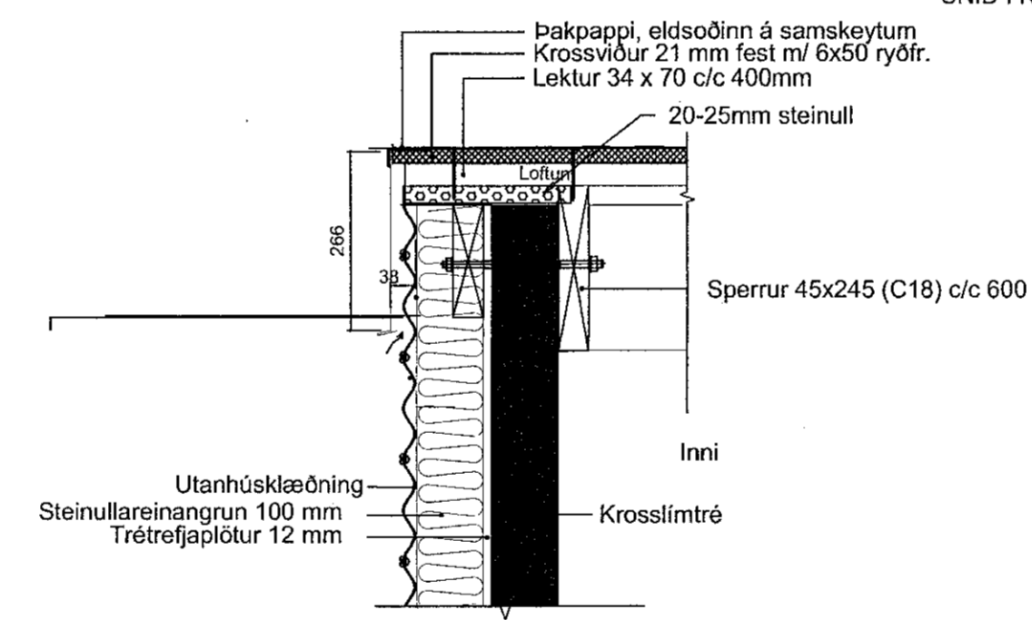
SNID Í GAFLVEGGI 1:10
