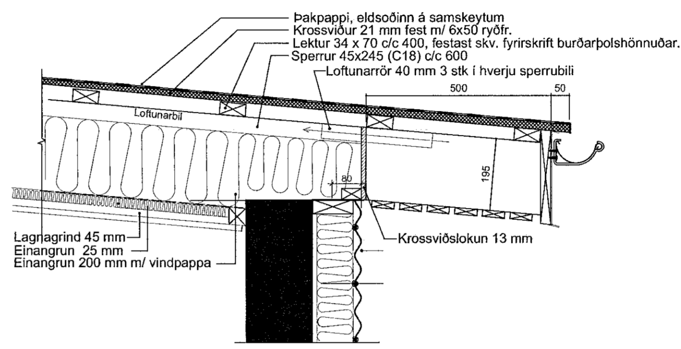
SNID Í NEDRI ÞAKKANT / RENUU 1:10
