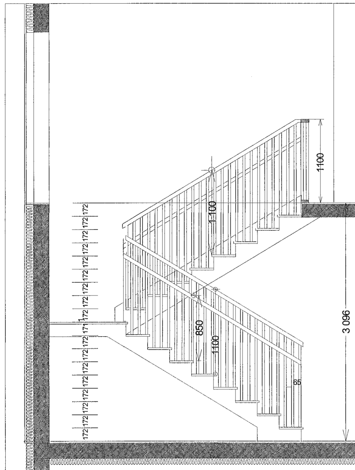
Stigi, Skurður 1:20
