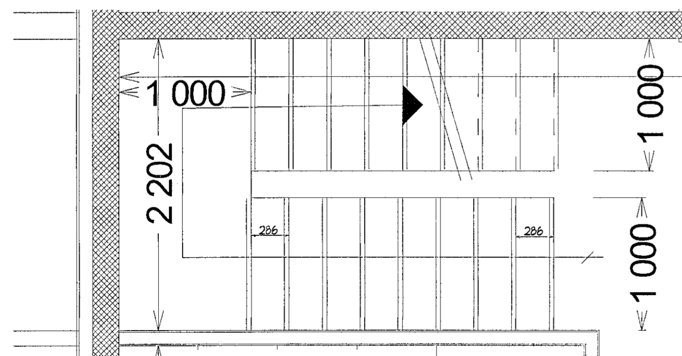
Stigi, Grunnmynd 1:20
