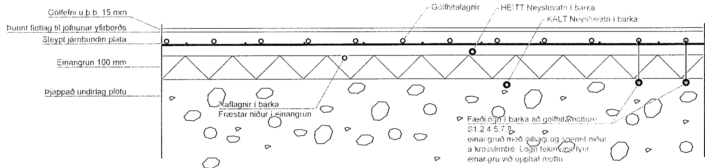
1 Frágangur lagna í gólfi neðri hæða 1:10
