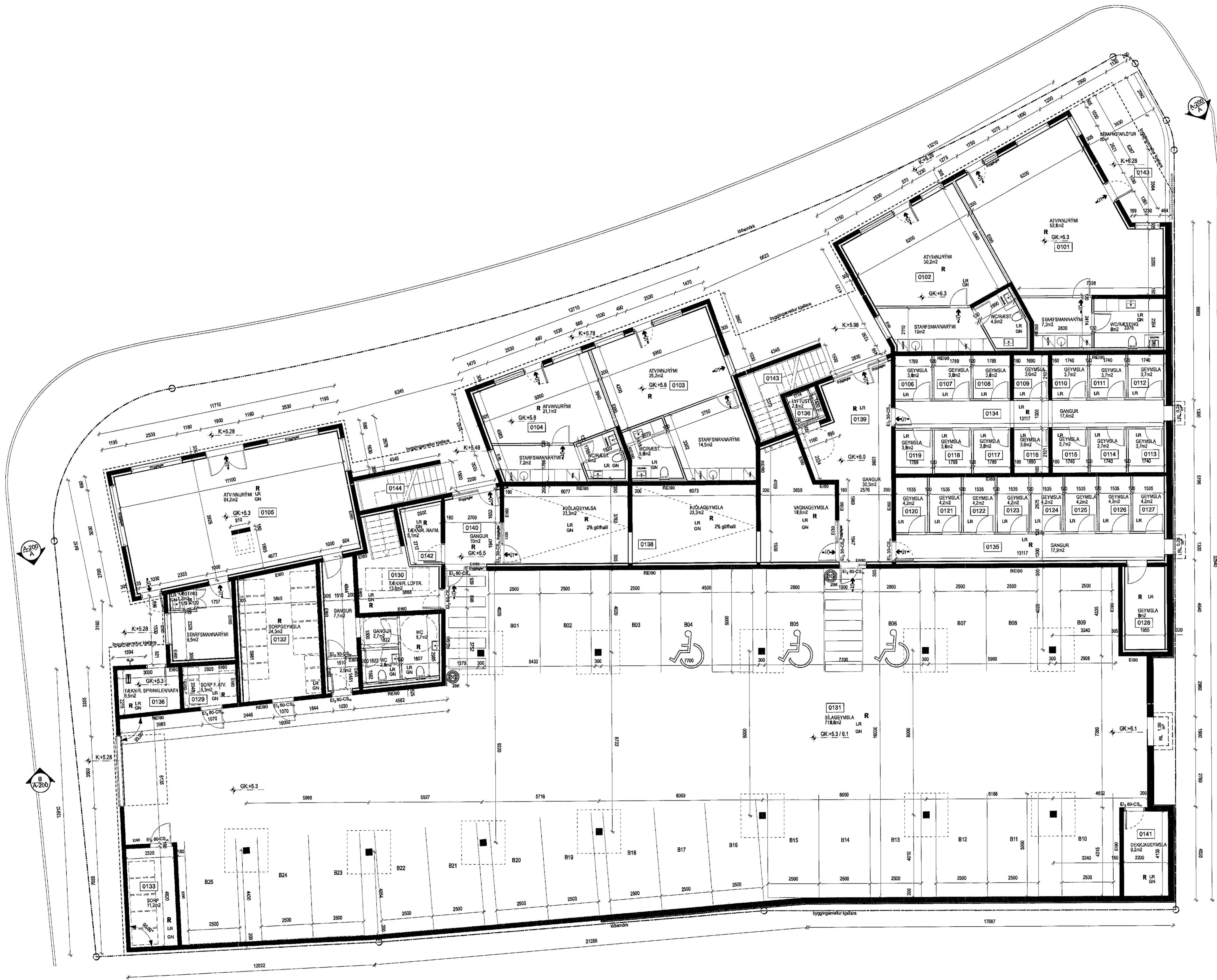
1 GRUNNMYND +1 Skali: 1:100
