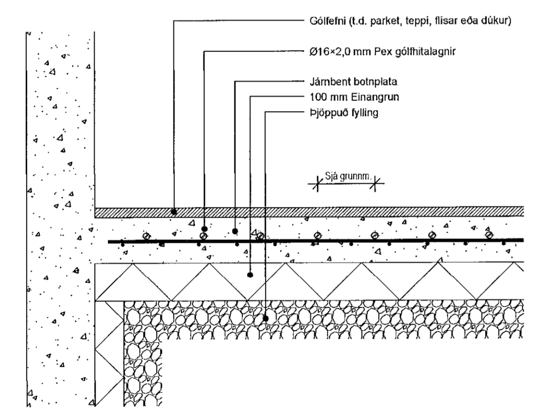
Sníð gólfhita í botnplötu 1:10
