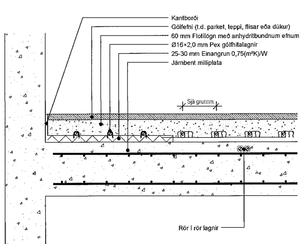
Sníð gólfhita í milliplötu 1:10
