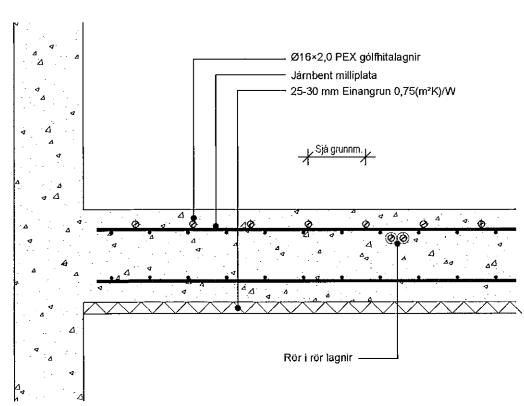
Sníð gólfhita í milliplötu bilskúrs 1:10
