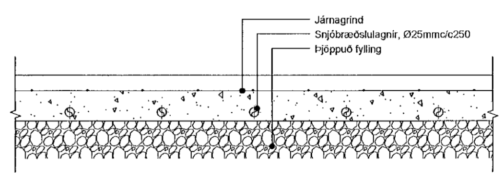
KENNISNIÐ SNJÓBRÆDSLÚ Í PLAN 1:10
