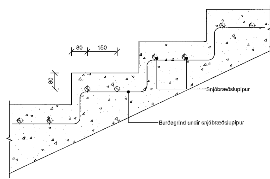
SNID Í TRÖPPUR 1:10
