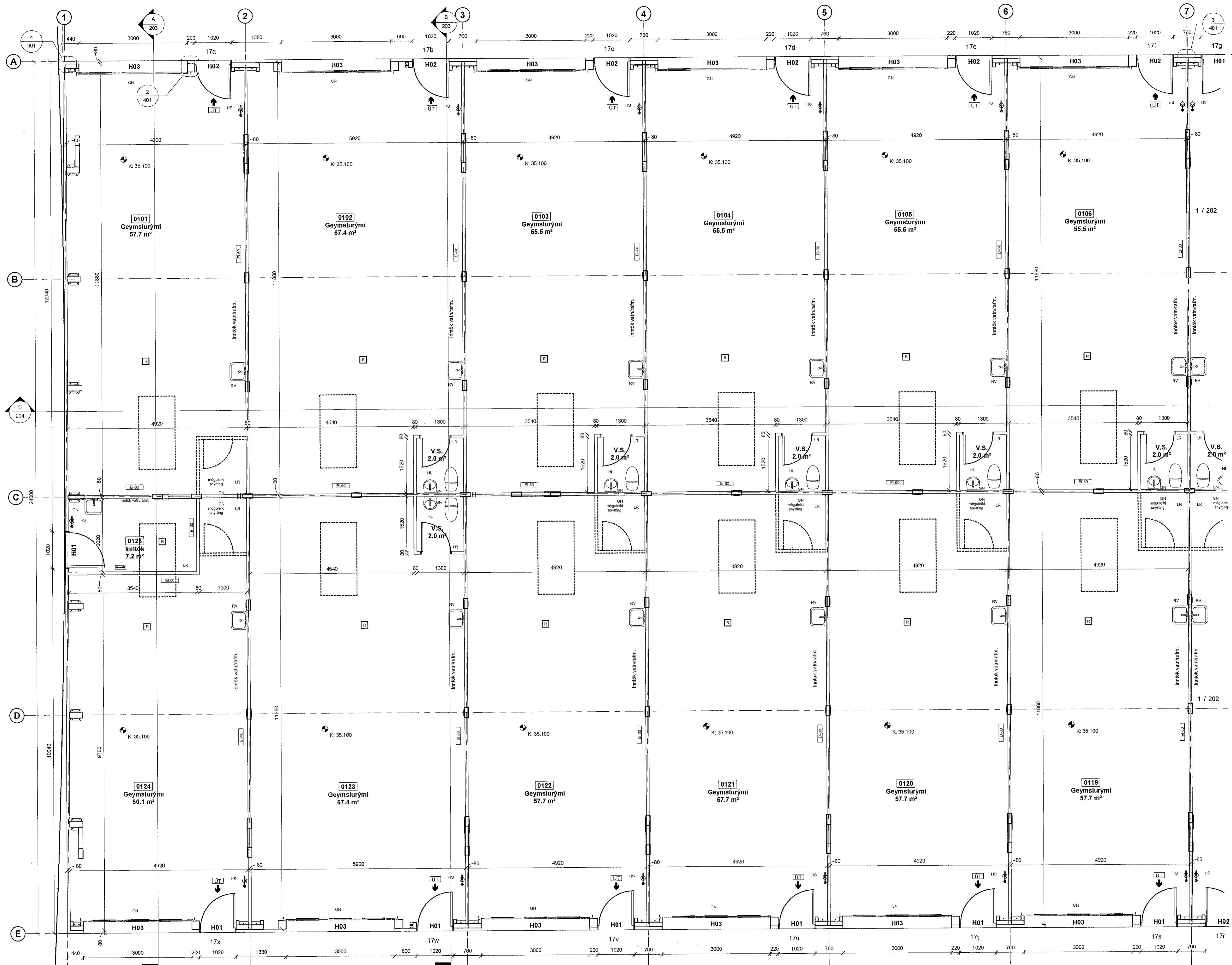
- GRUNNMYND 1.HÆÐ - Hluti 1-7 1 : 50
