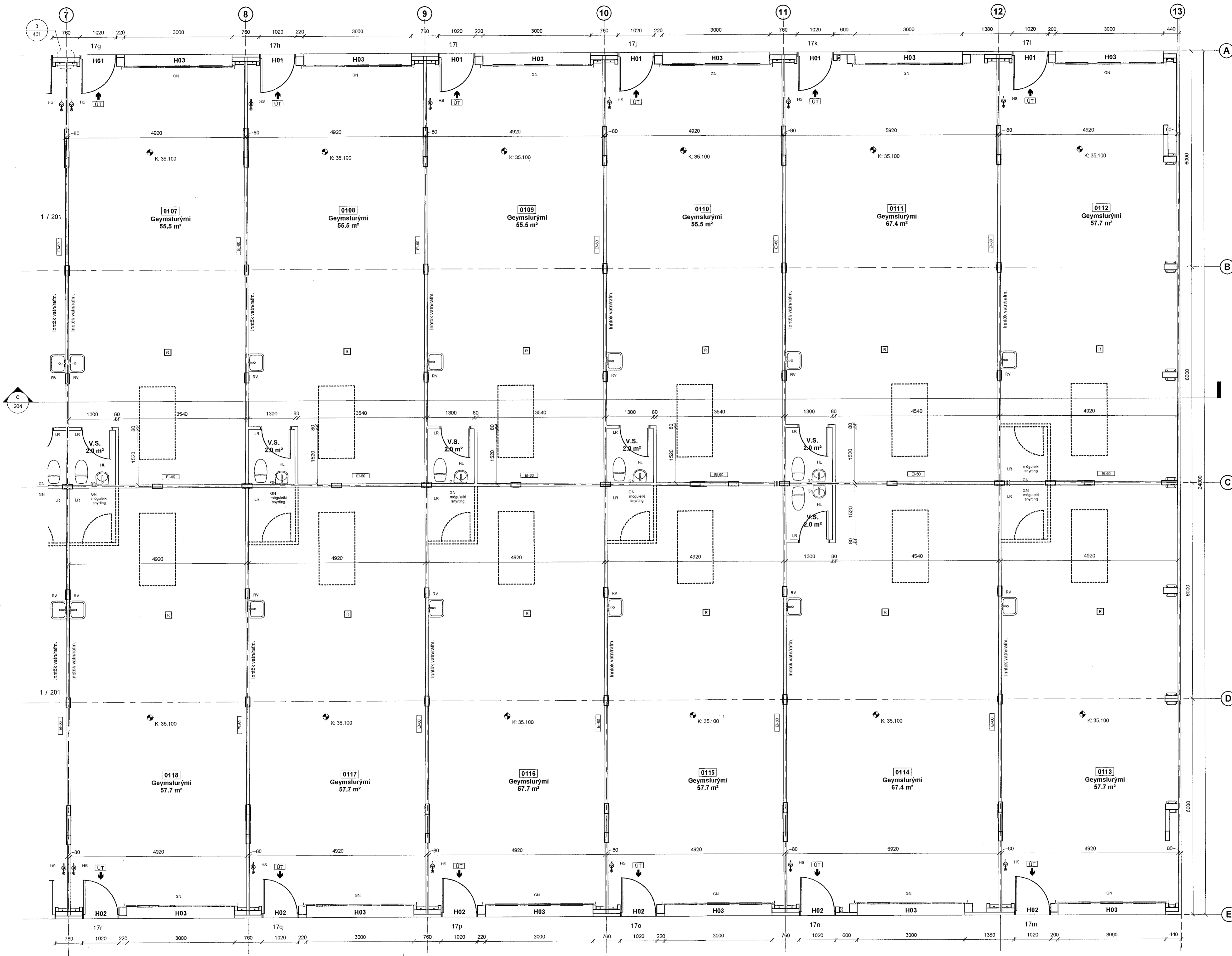
- GRUNNMYND 1.HÆÐ - Hluti 7-13 1:50
