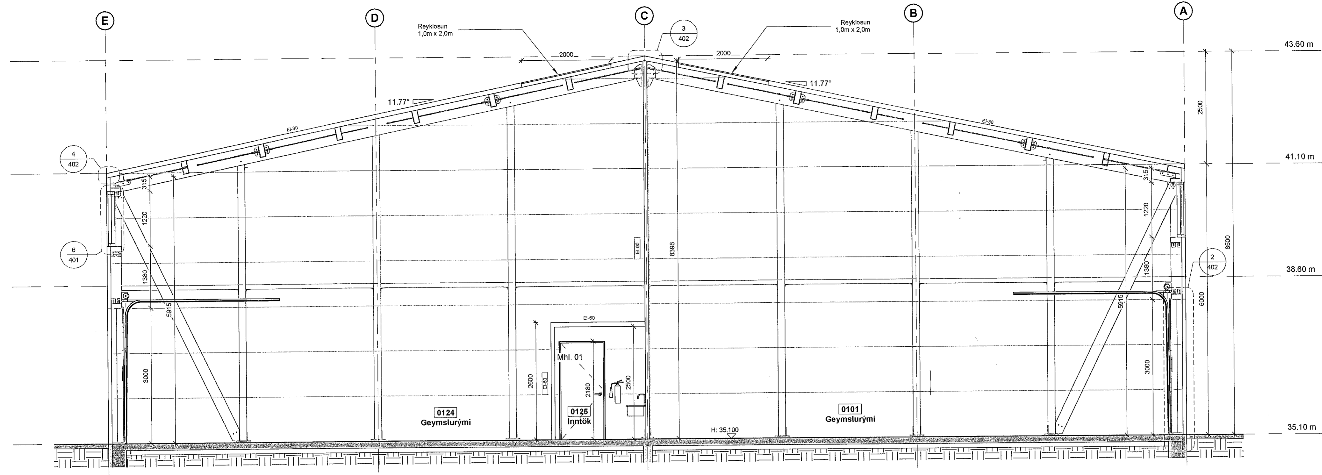
- SNID A 1 : 50
