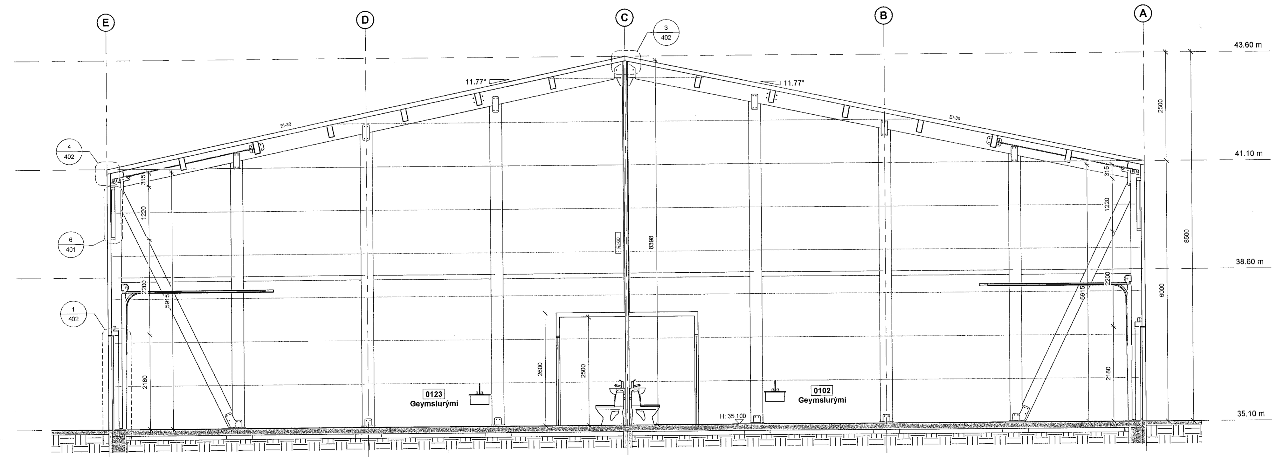
- SNID B 1 : 50
