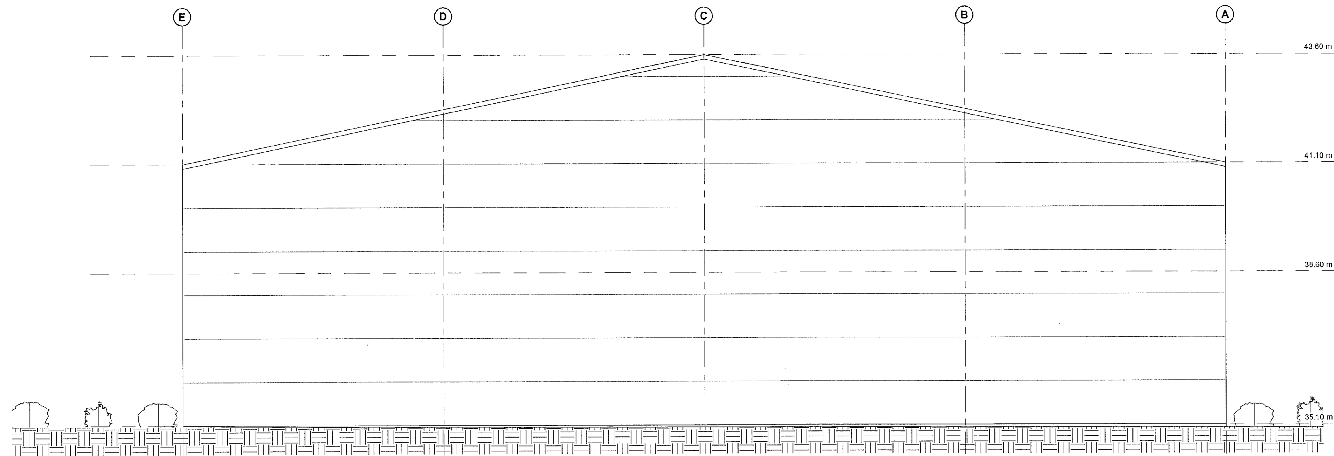
- NORÐAUSTUR 1 : 50
