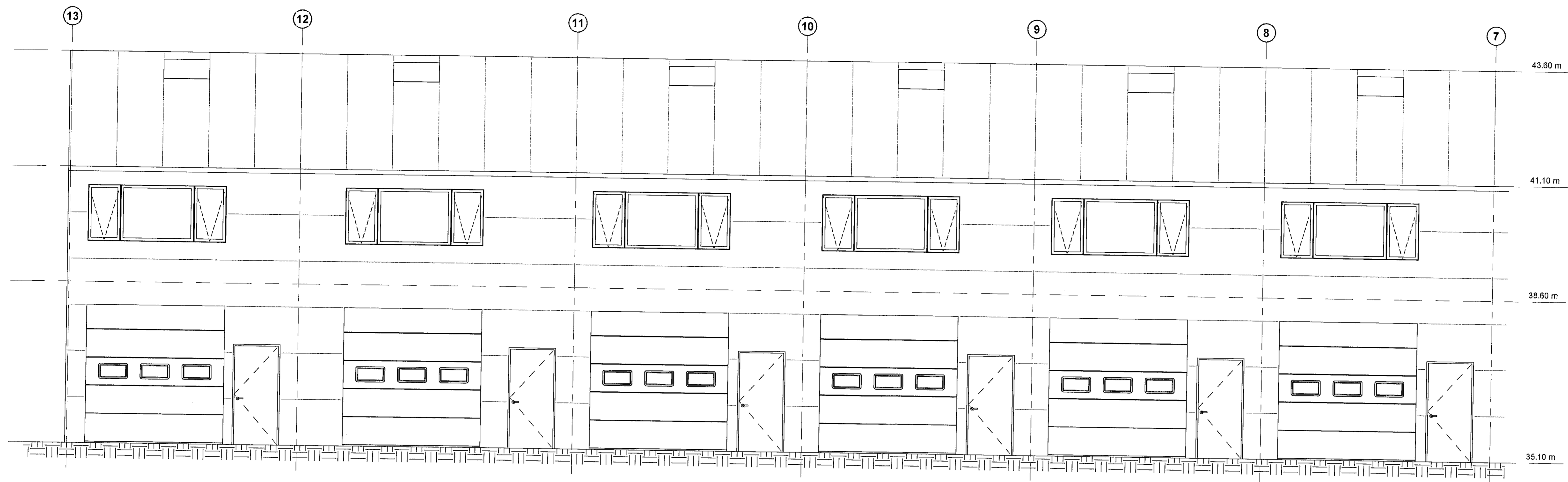
- NORÐVESTUR - Hluti 7-13 1:50
