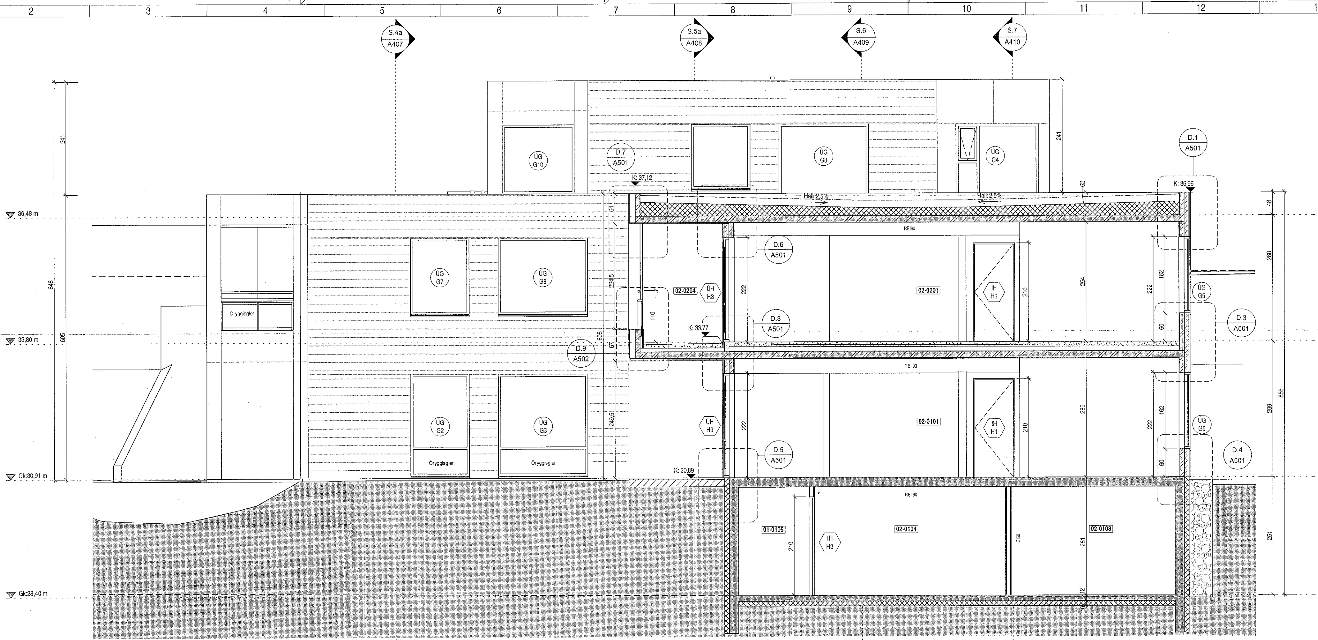
Snið 1. MHL.02 1 : 50
