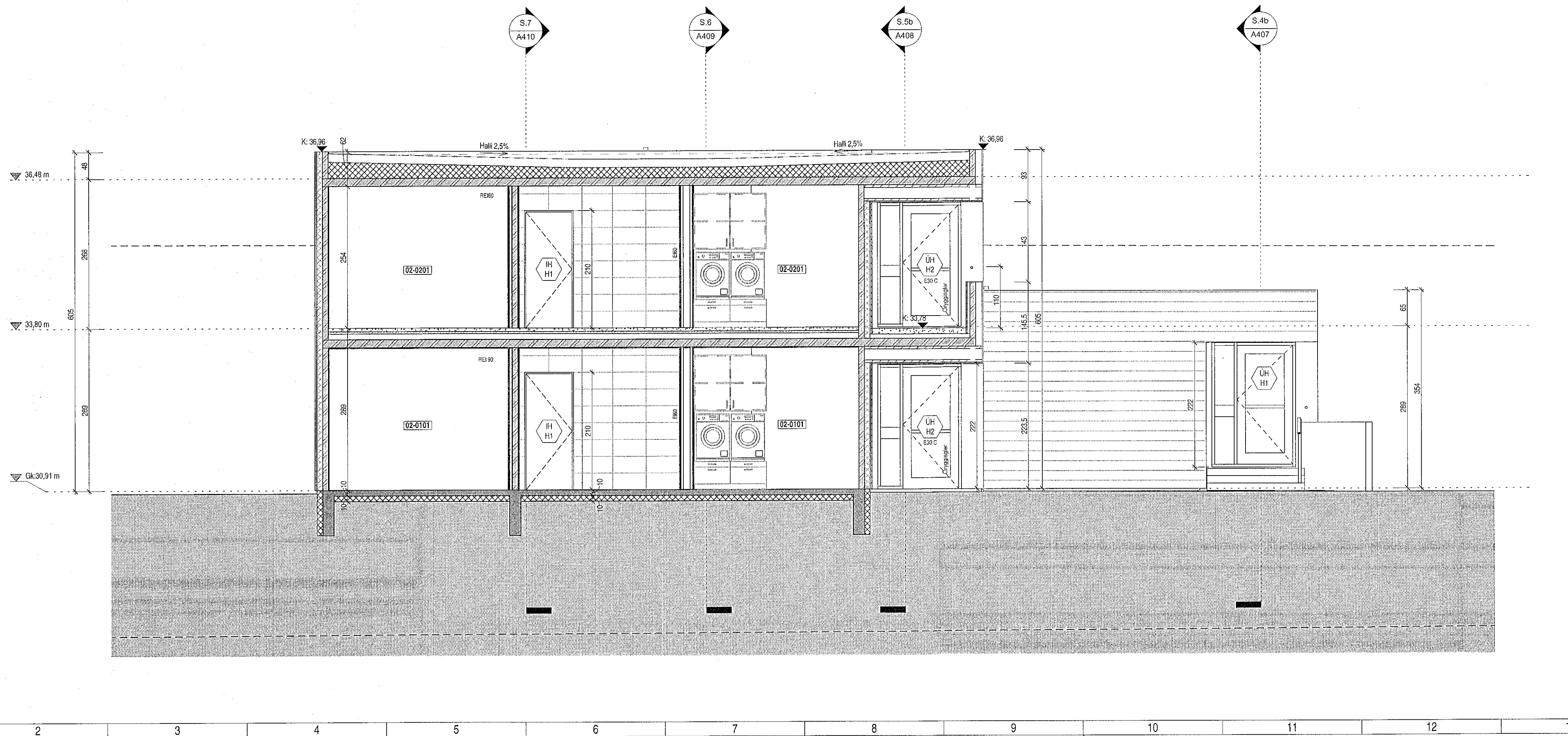
Snið 2. MHL.02 1 : 50
