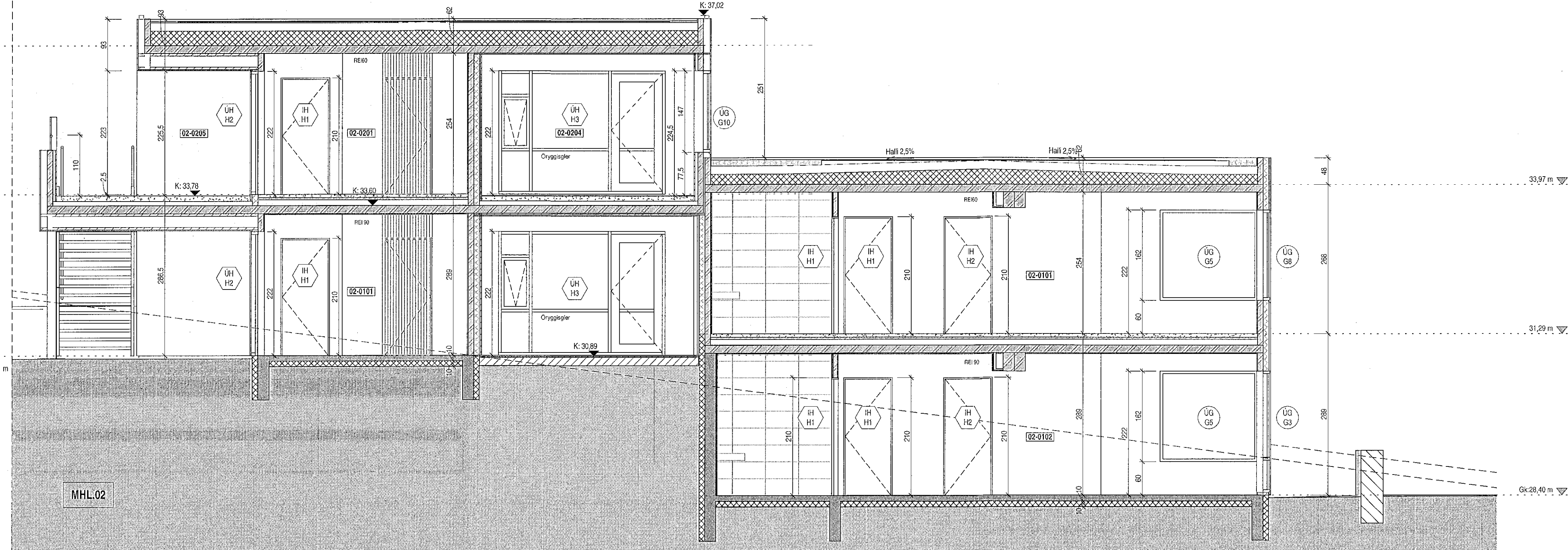
Snið 5b 1:50
