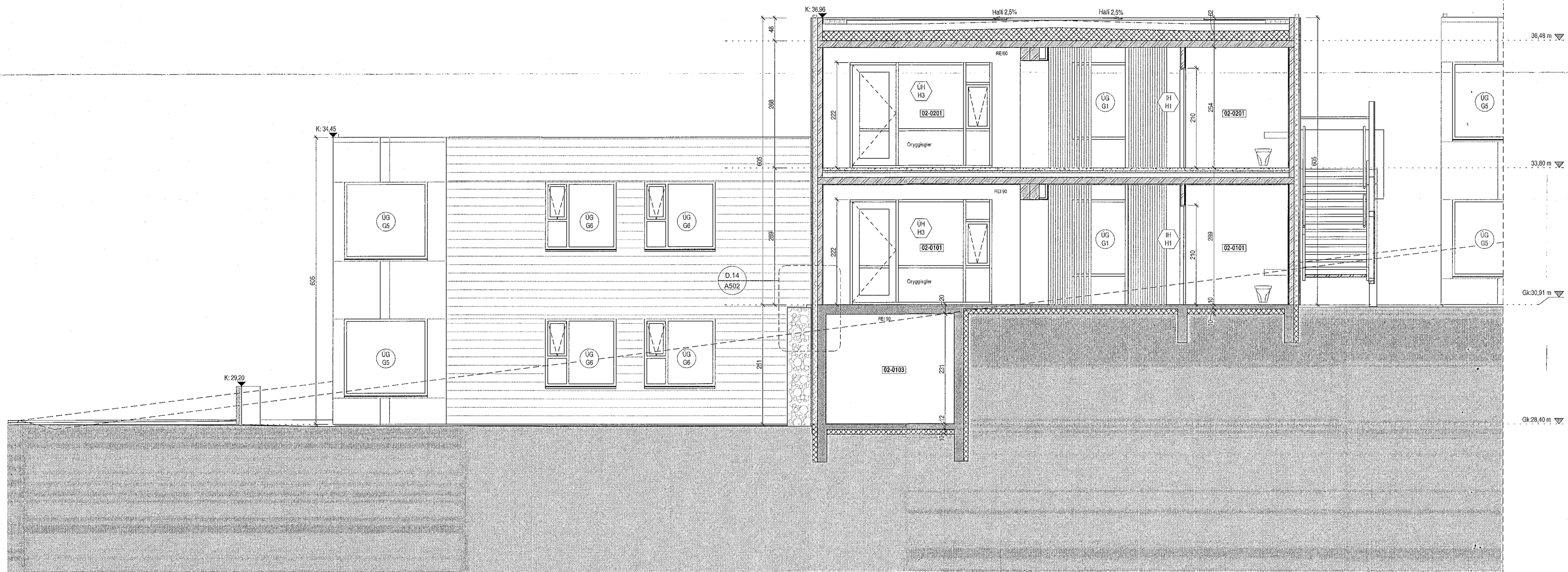
Snið 7 1:50
