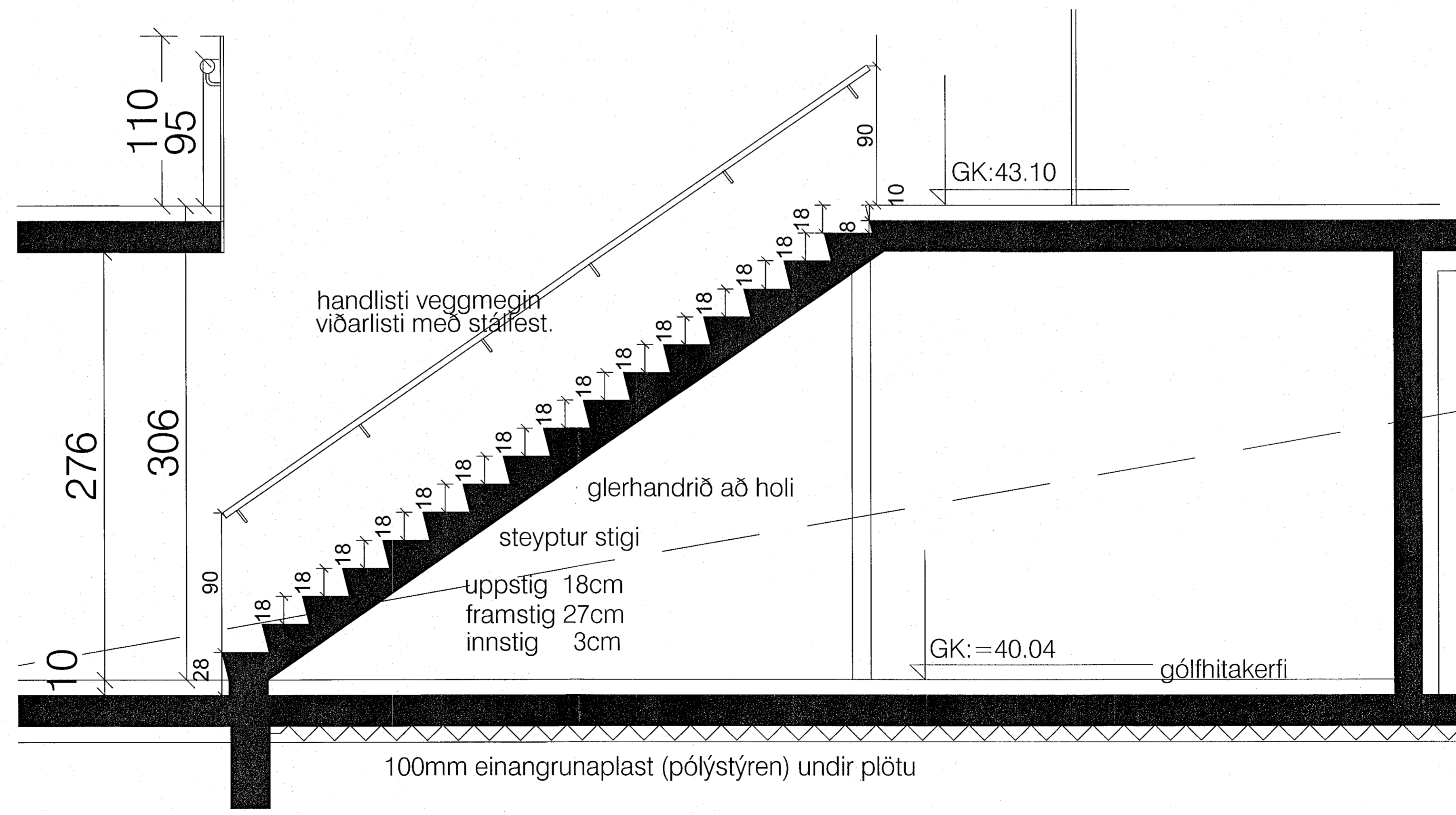
sneiðing í stiga 1:20
