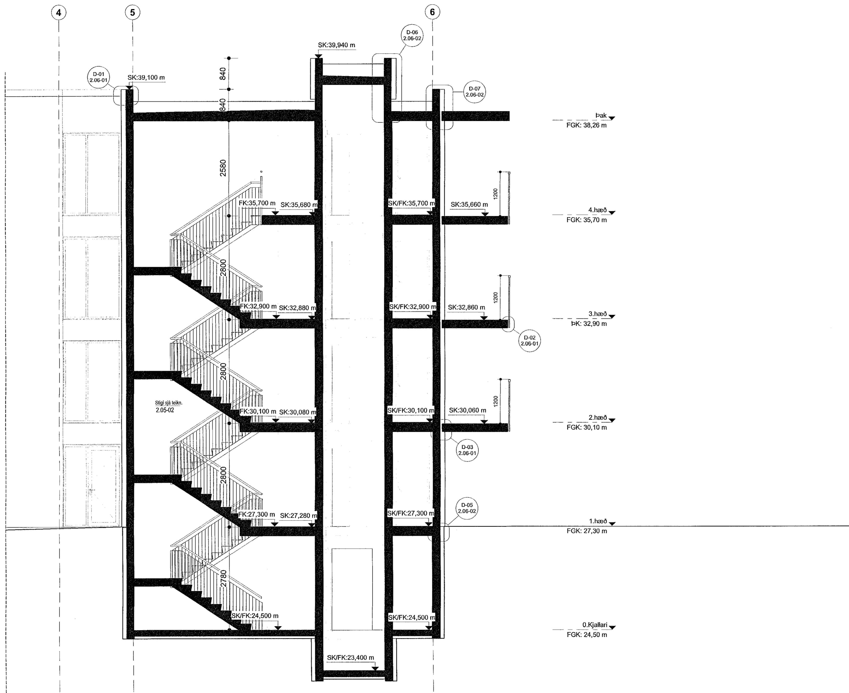
Snið B-B
