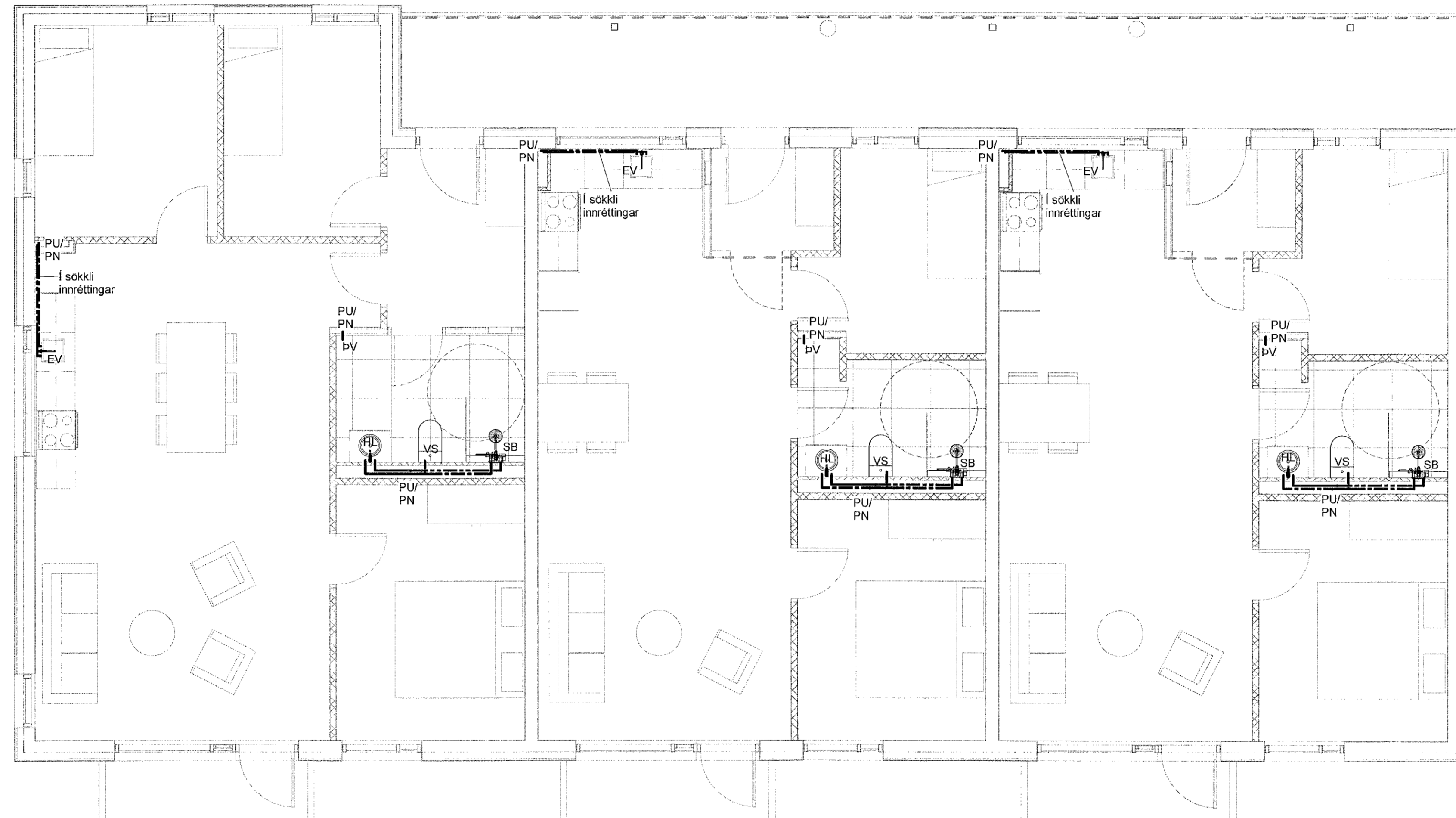
1 2. hæð - 1 1 : 50
