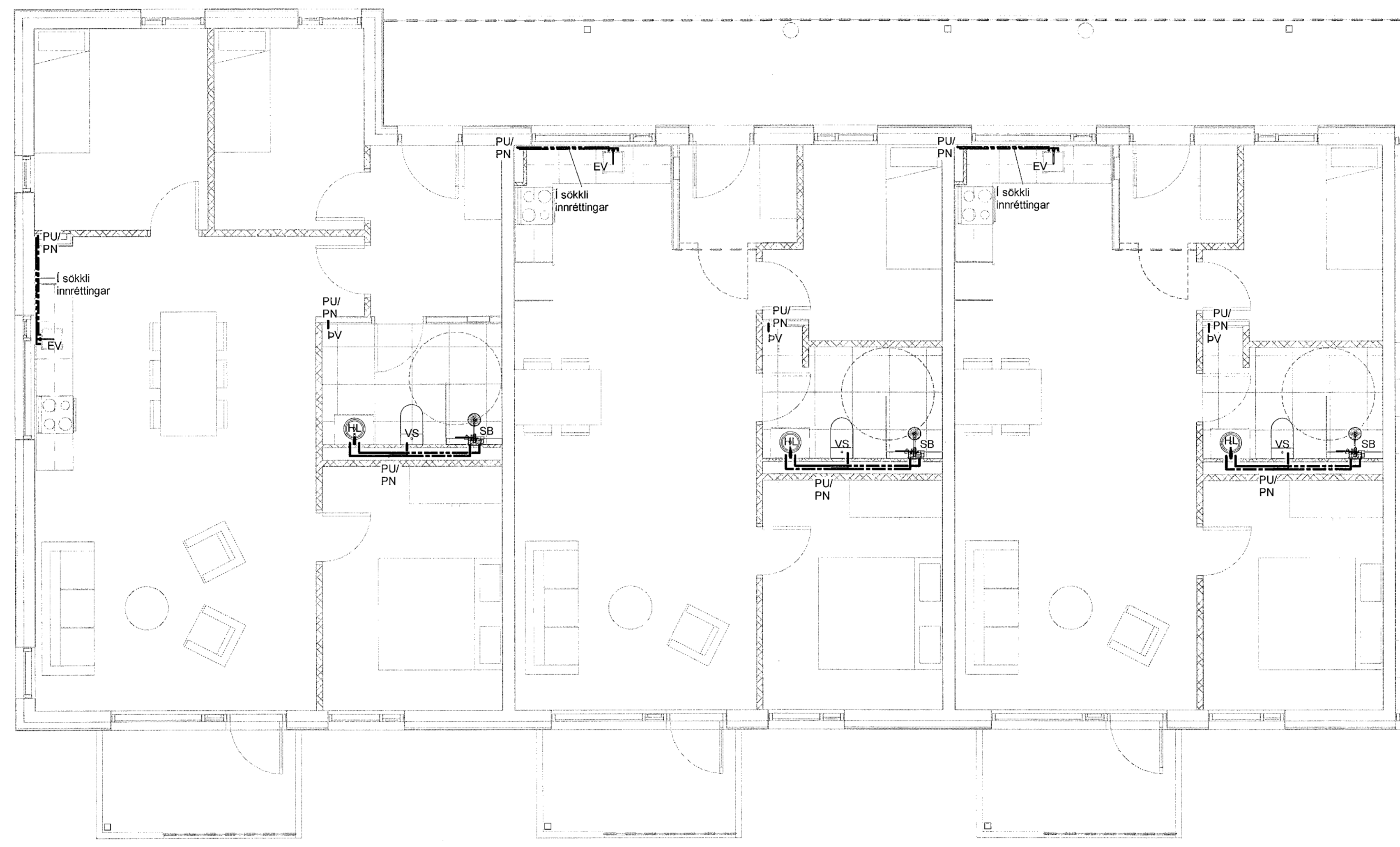
1 3. hæð - 1 1 : 50
