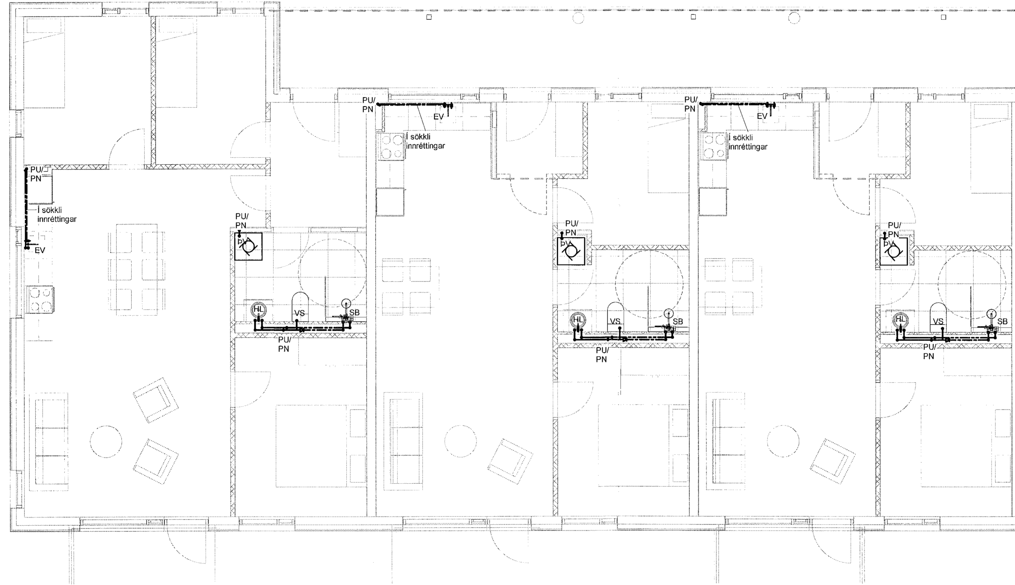
1 4. hæð - 1 1 : 50
