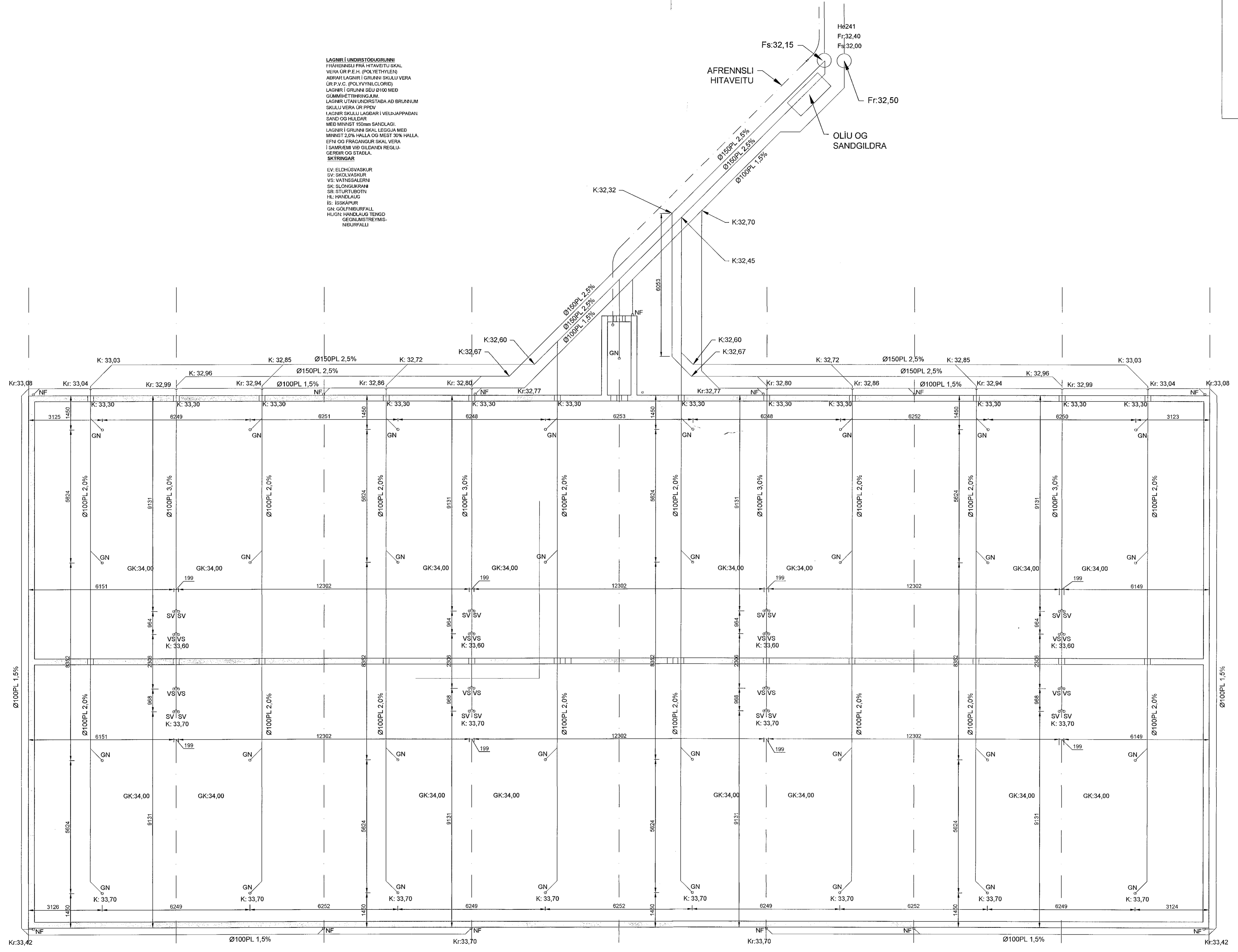
FRÆRENNSLISLAGNIR - GRUNNMYND 1:75 (A2)
