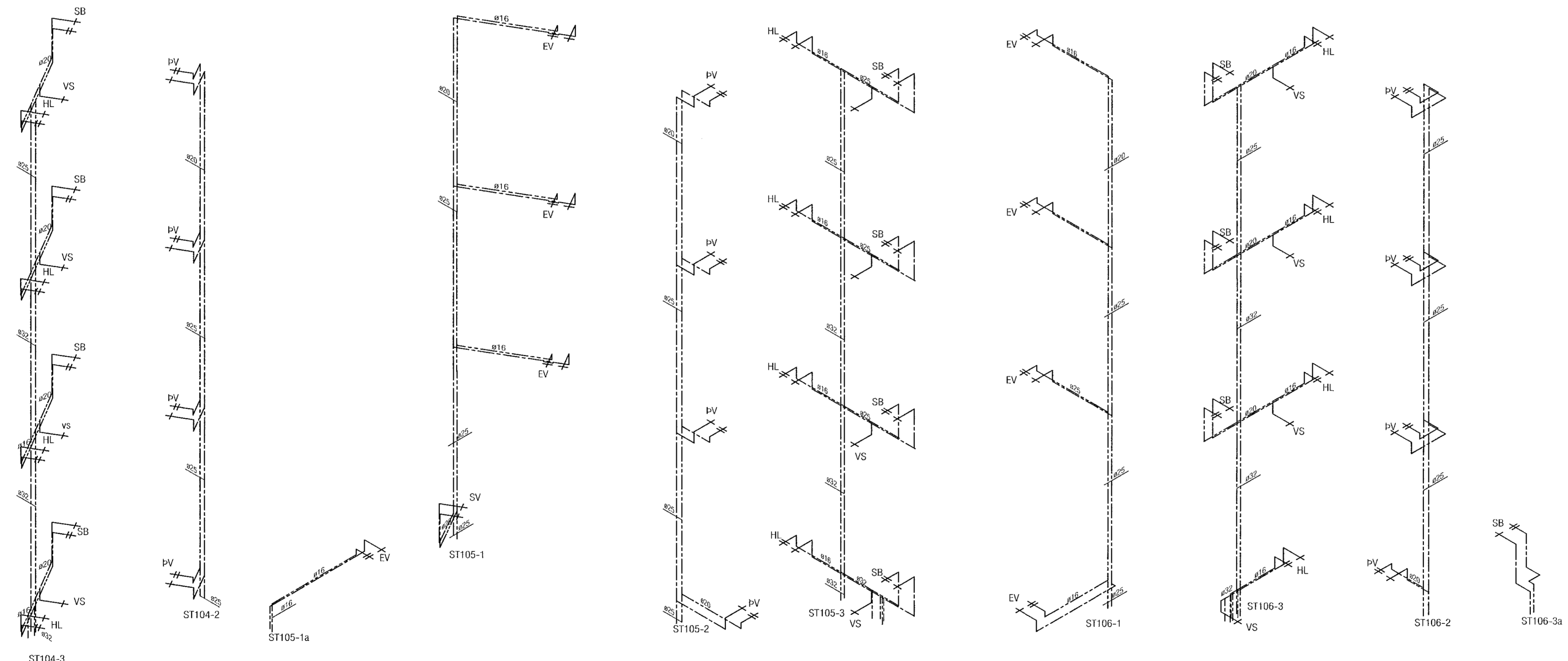
RÚMMYND NEYSLUVATNSLAGNA LAGNIR ERU PE-X, AL/PEX EDA PP-R, SJA SKÝRINGAÐLAD L-01
