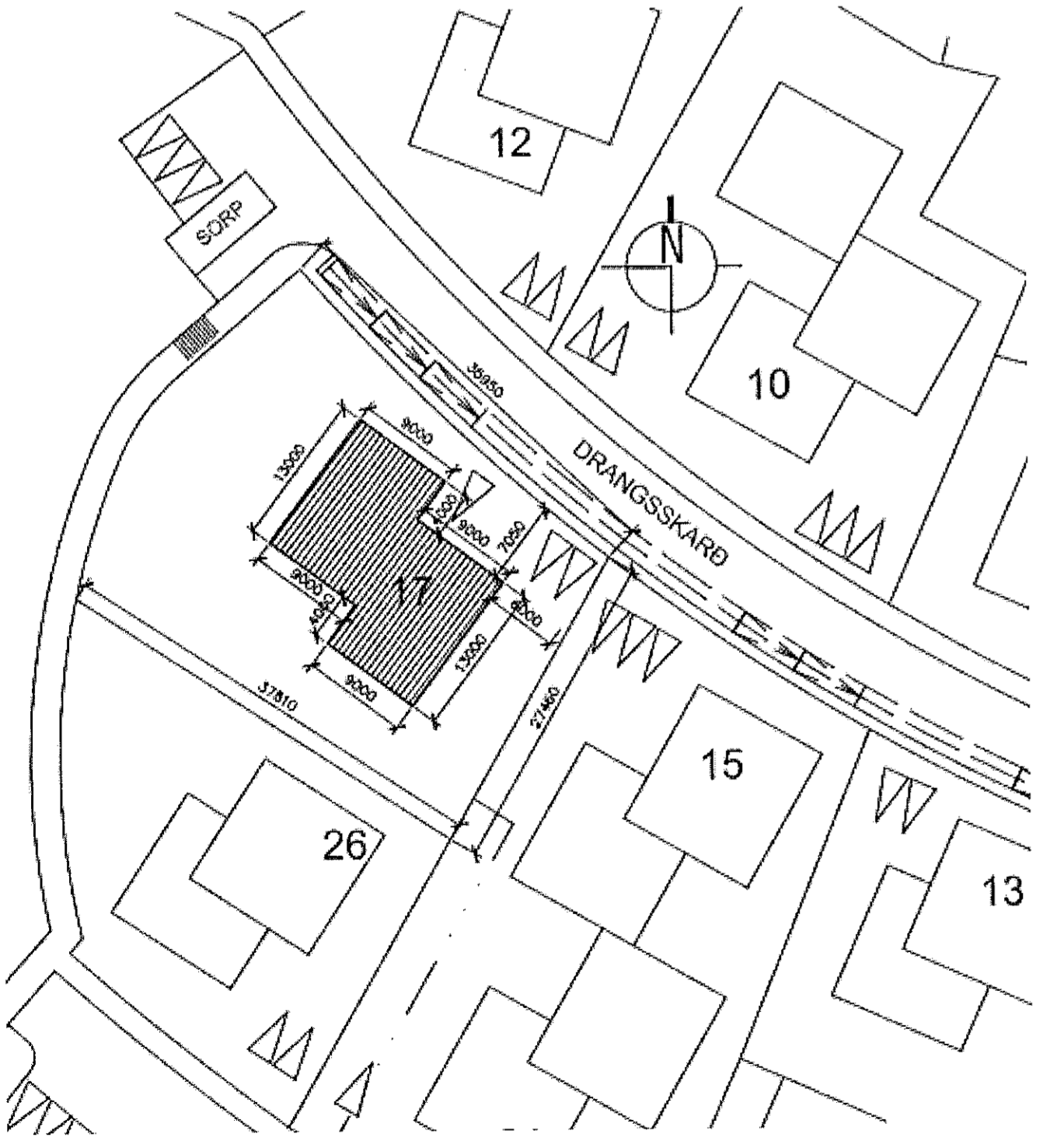
2 Afstöðumynd 1:500
