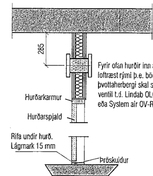
Loftun f. baðh og þvottah. Rist fyrir ofan hurð eða rífa undir hurð. 1:20
