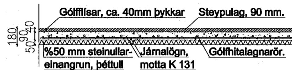
Gólf sólstofu, snið.
