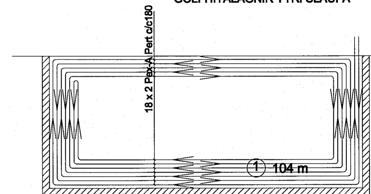
GÓLFHITALAGNIR YTRI SLAUFU
