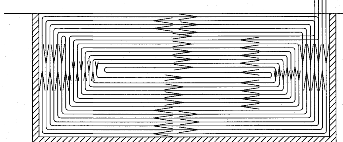
GÓLFHITALAGNIR, GRUNNMYND, BÁÐAR SLAUFUR.
