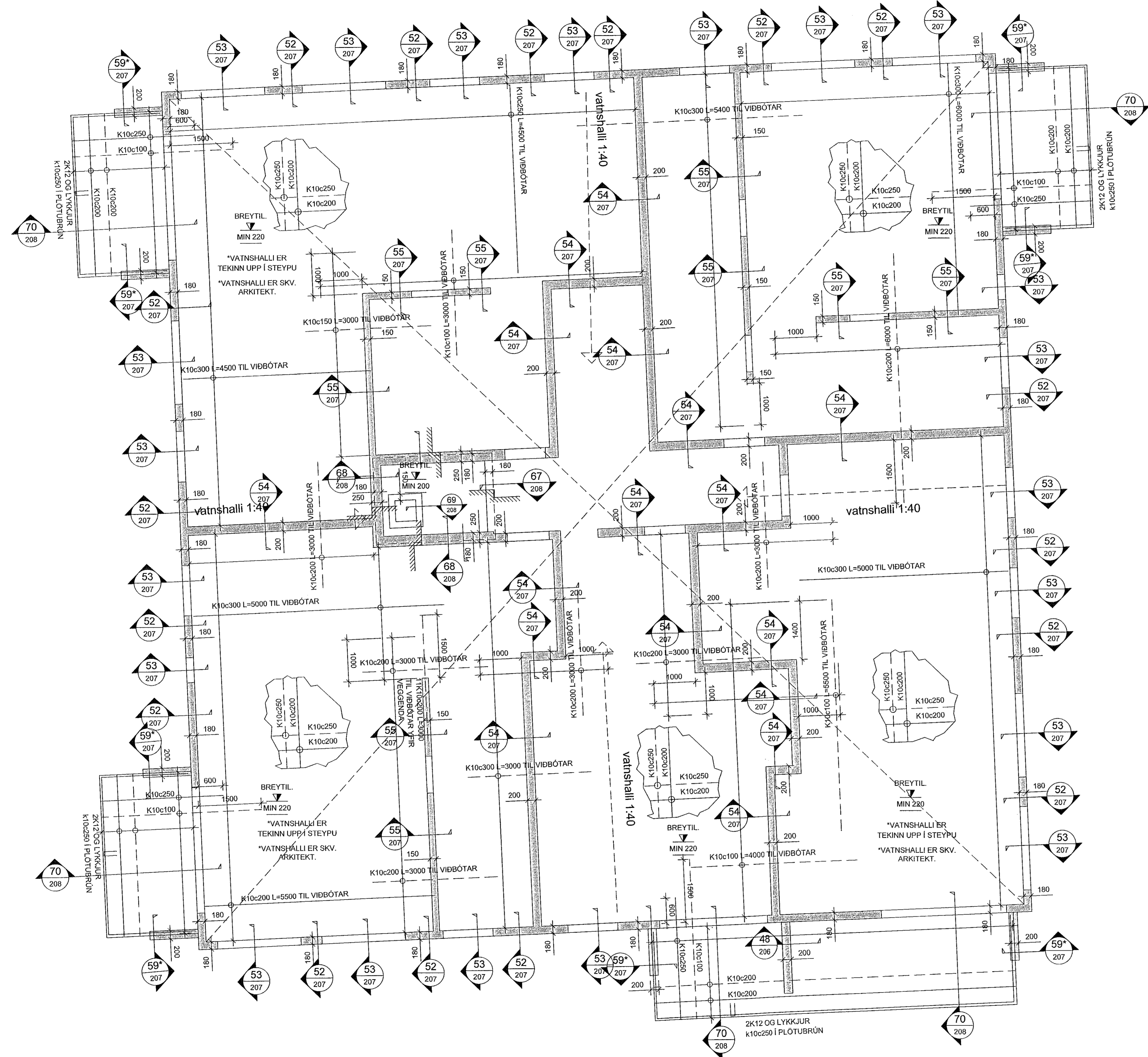
VEGGIR OG LOFTAPLATA 3.HÆÐAR, GRUNNMYND MKV. 3
