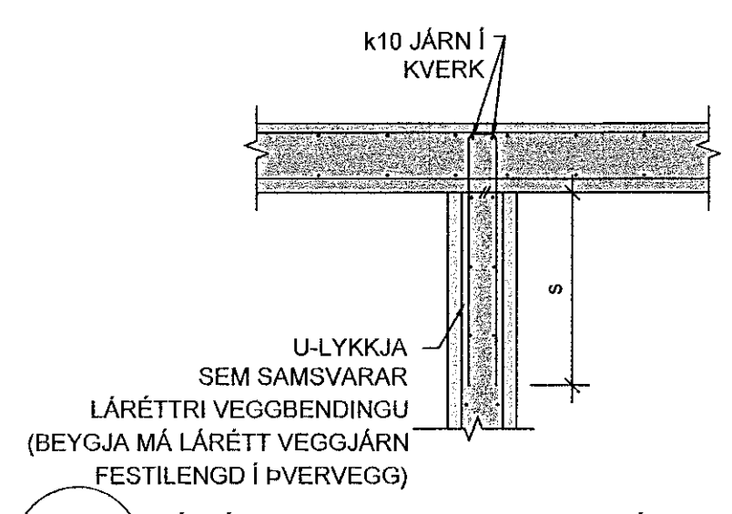
K4 LÁRÉTT KENNISNIÐ - VEGGMÓT Mkv. 2
