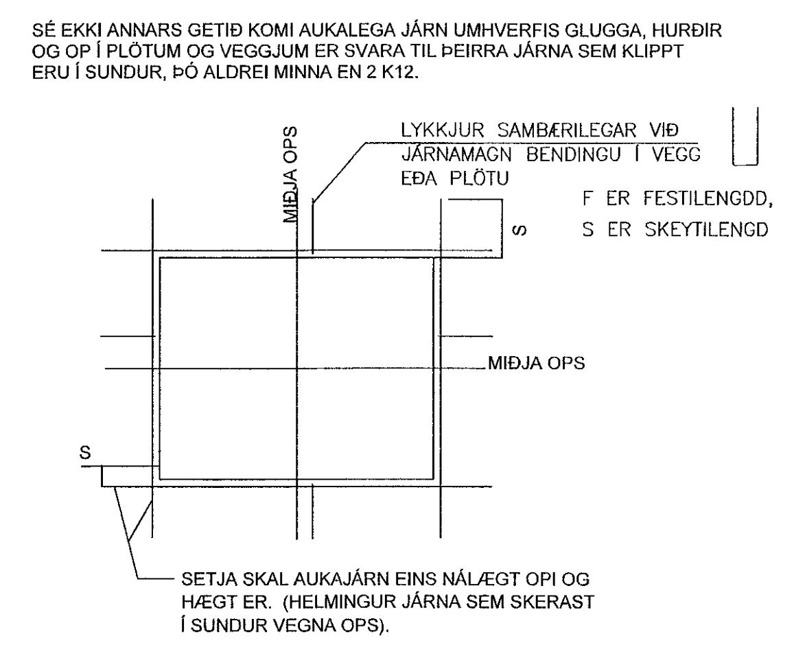
K6 JÁRNUN KRINGUM OP Mkv. 2
