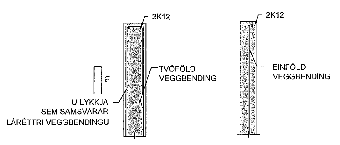
K5 LÁRÉTT KENNISNIÐ - VEGGENDI TVÖFÖLD BENDING OG EINFÖLD VEGGBENDING Mkv. 2
