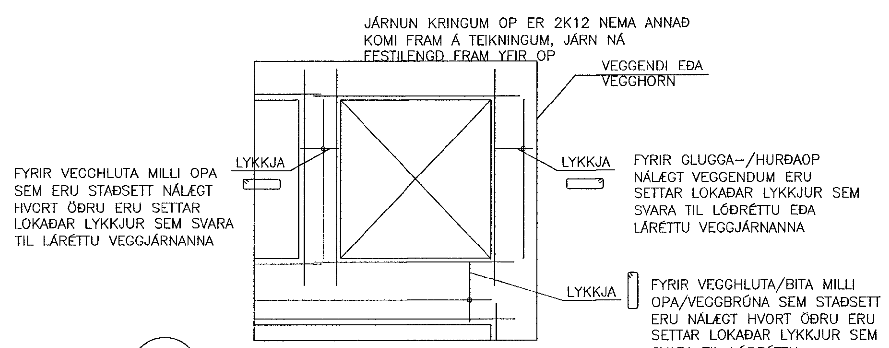
K0 ÁSYND Á VEGG - JÁRNUN VEGGHLUTA Mkv. 2
