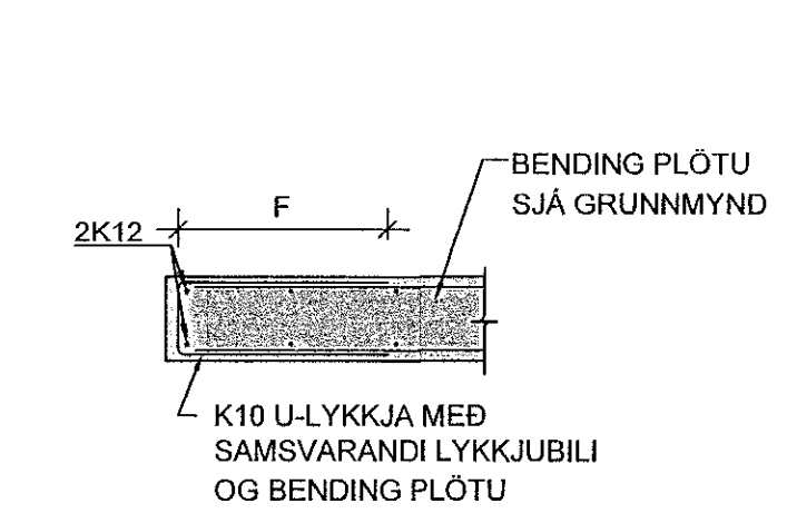
K2 LÓDRÉTT KENNISNIÐ - PLÖTUBRÚN Mkv. 2
