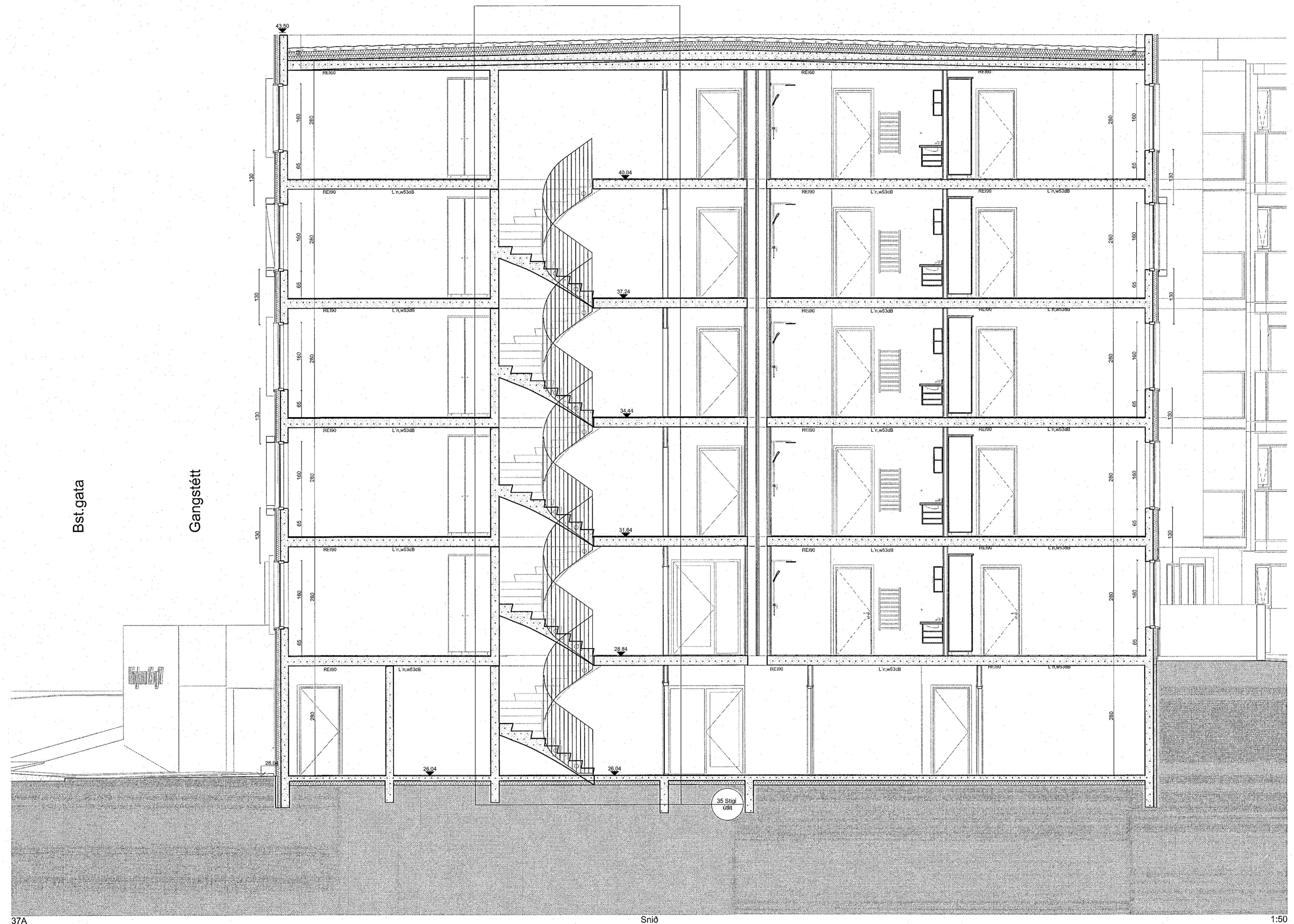
37A Sníð 1:50
